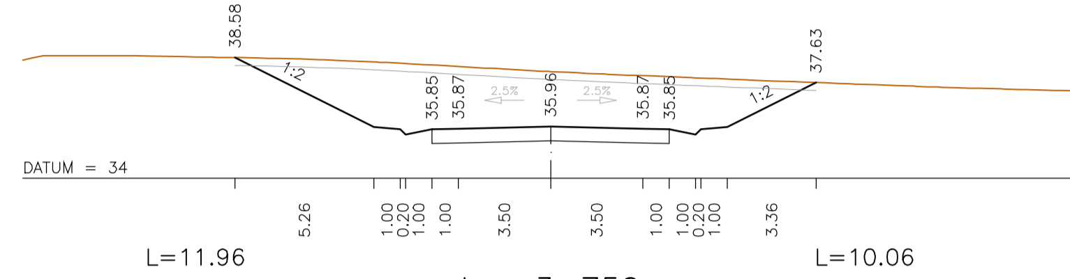
km=3+750
