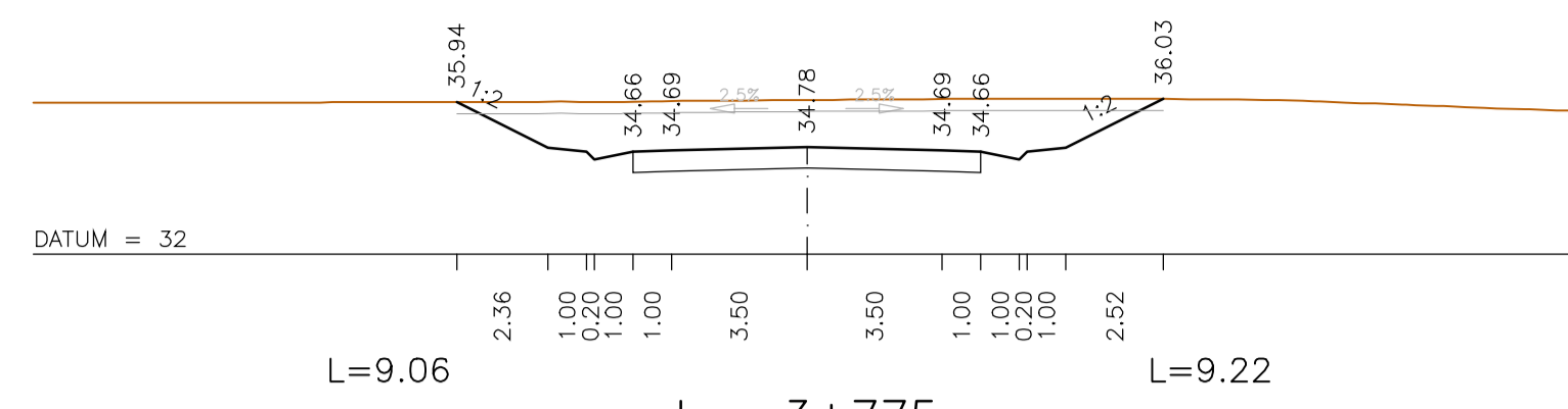
km=3+775
