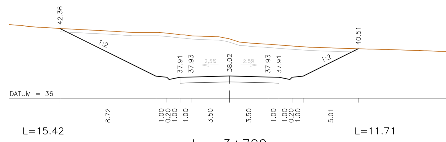
km=3+700
