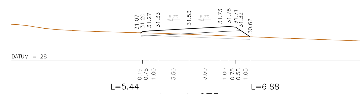
km=4+075
