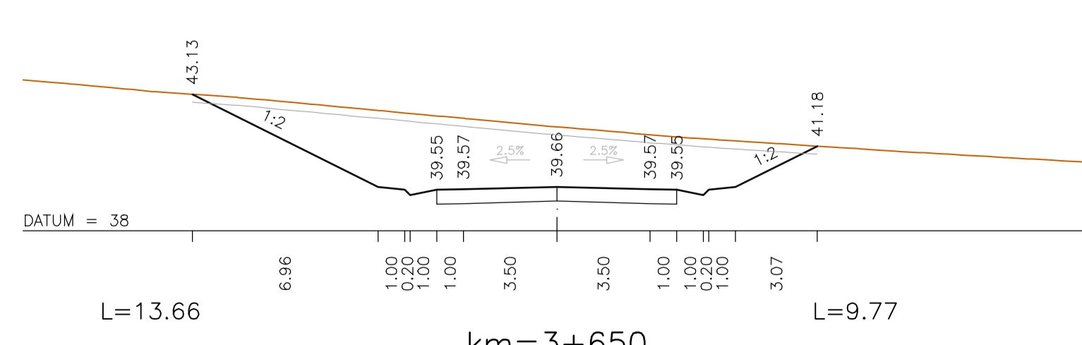
km=3+650
