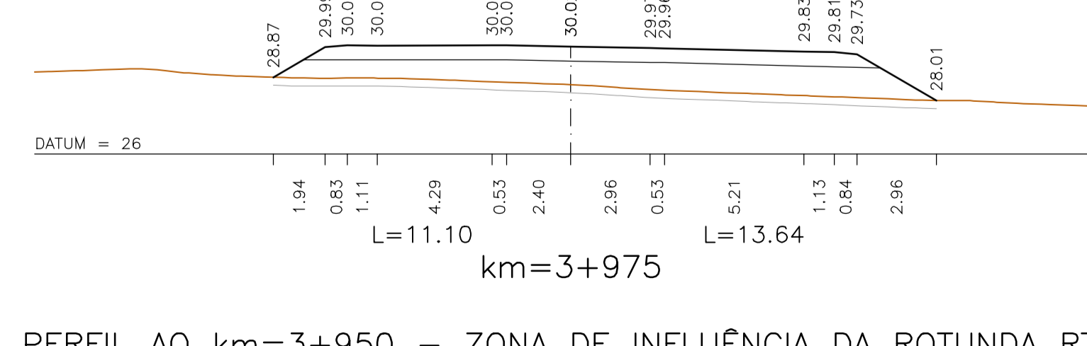
km=3+975
