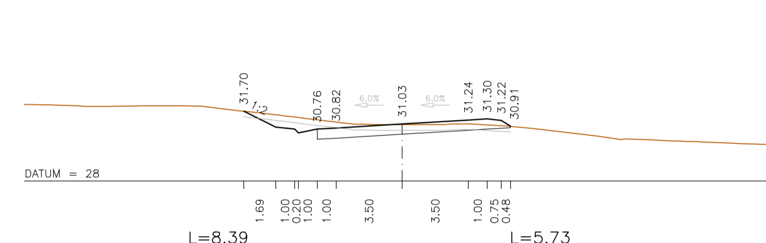
km=4+050
