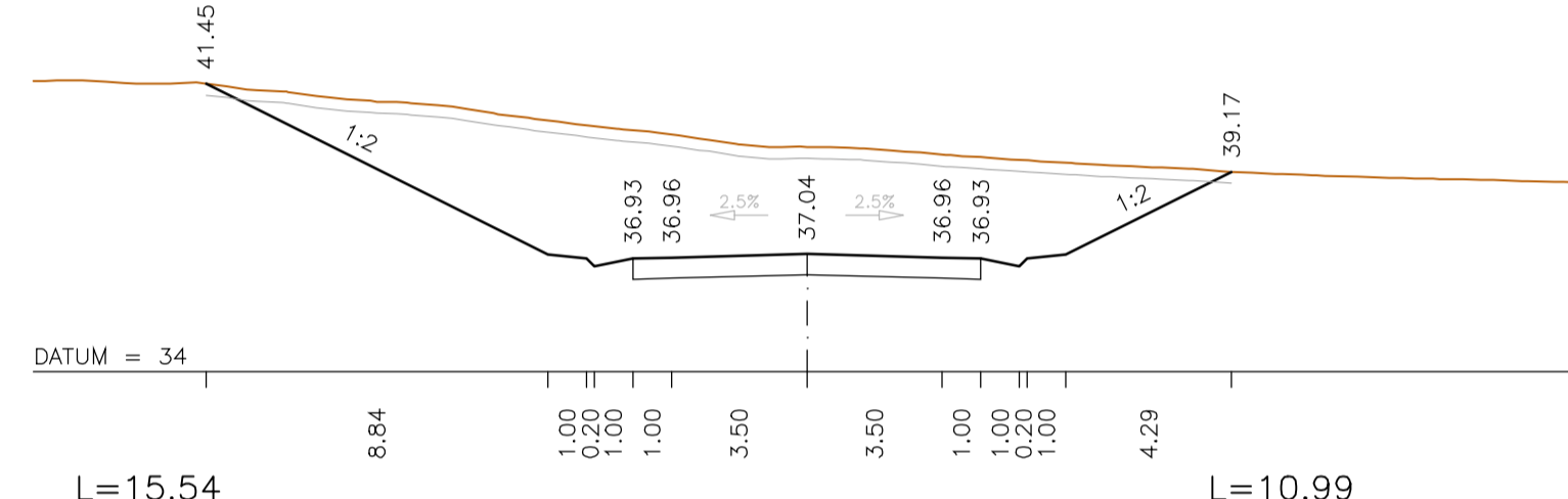
km=3+725
