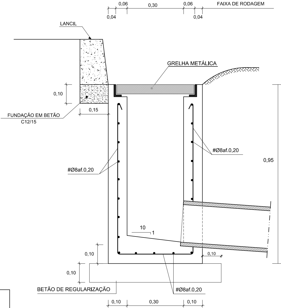
CORTE A-A
