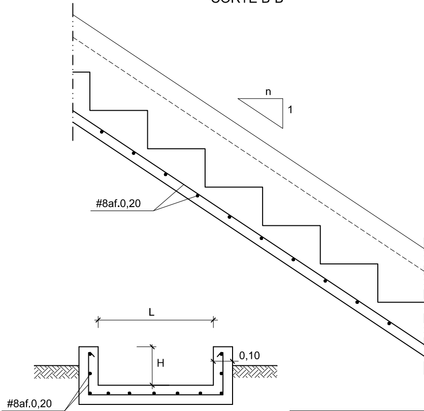
CORTE B-B
