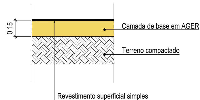
SOLUÇÃO DE PAVIMENTO SC3-B Restabelecimentos não pavimentados com inclinação superior a 10% Esc. 1:20
