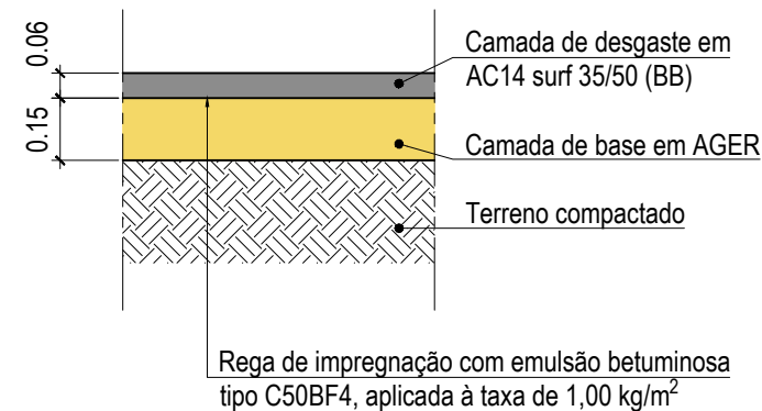
SOLUÇÃO DE PAVIMENTO SC2 Restabelecimentos pavimentados Esc. 1:20
