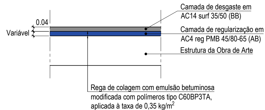
SOLUÇÃO DE PAVIMENTO SC4 Passagens Superiores Esc. 1:20
