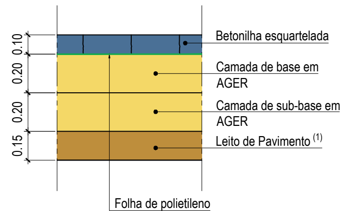
SOLUÇÃO DE PAVIMENTO SC1 Betoniha esquadrelada Esc. 1:20
