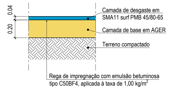
SOLUÇÃO DE PAVIMENTO SC5 Serventias pavimentadas Esc. 1:20
