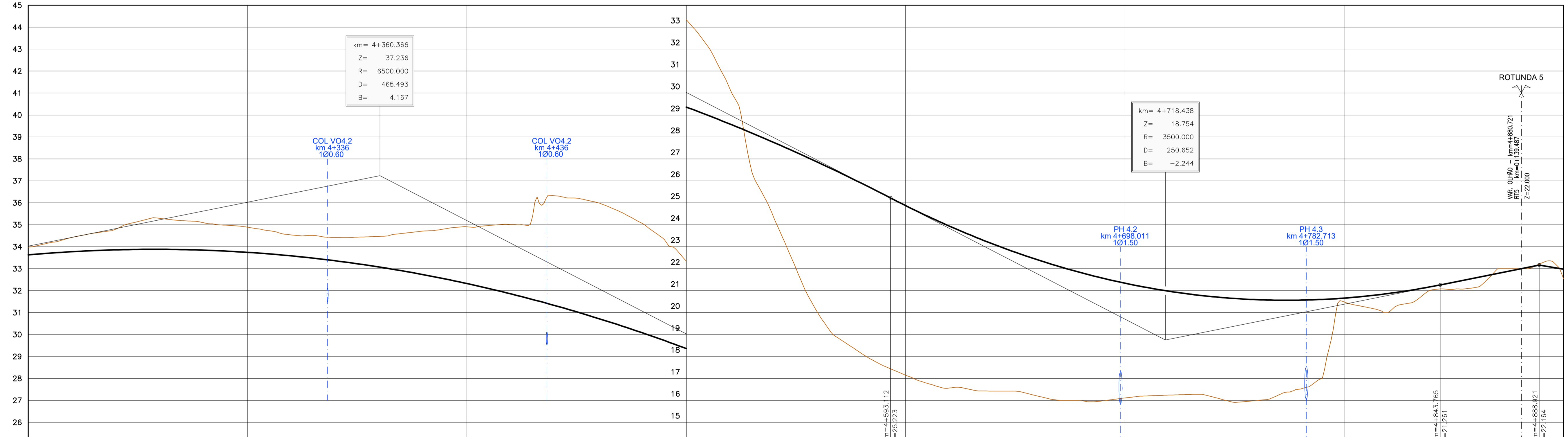
EN125 - VARIANTE DE OLHÃO PERFIL LONGITUDINAL Esc. H=1:1000 V=1:100
