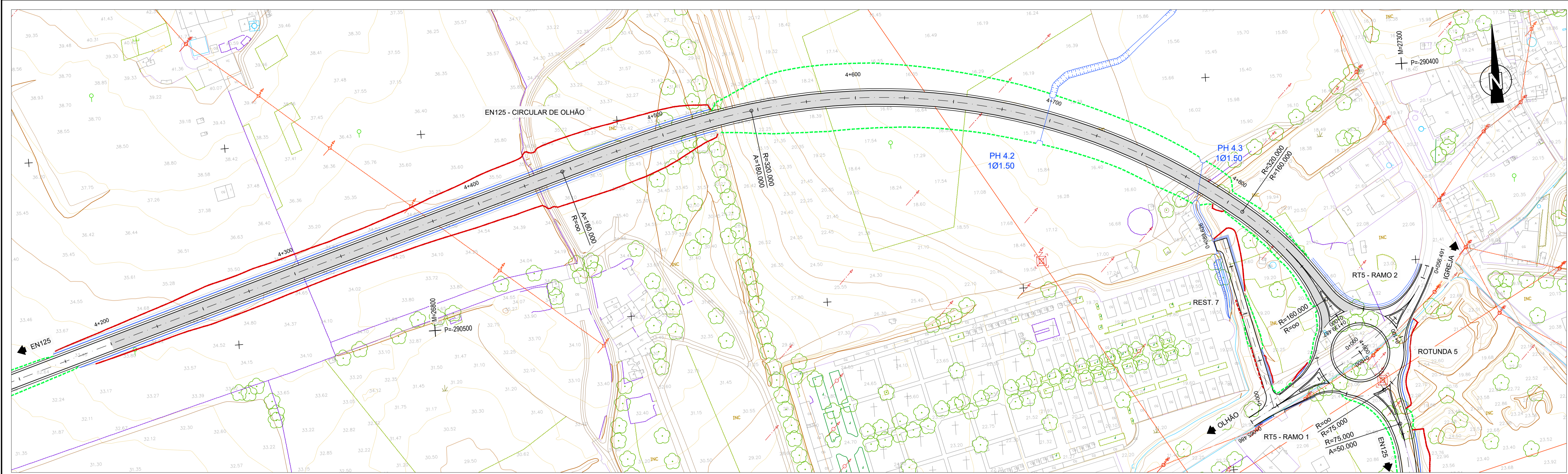
PLANTA Esc. 1:1000
