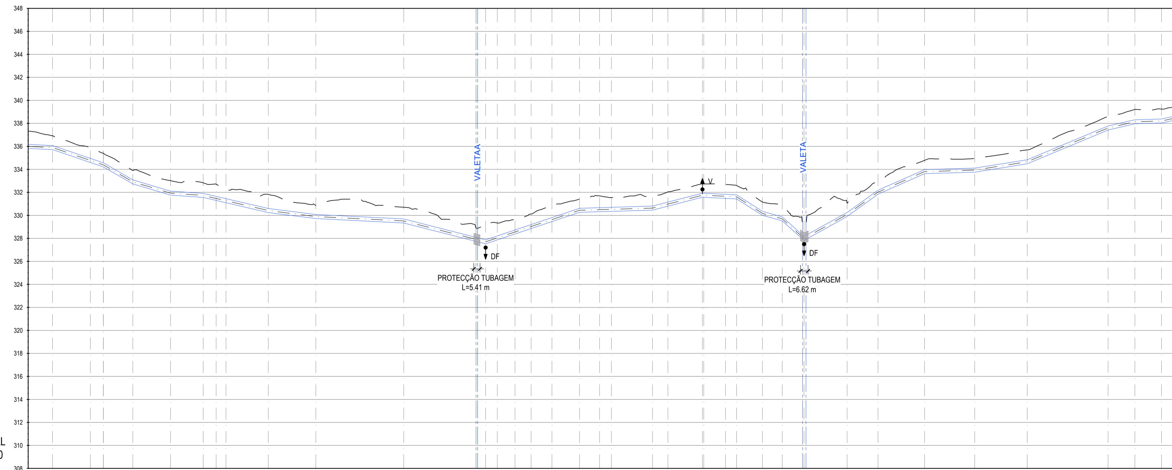
15000.00 a 16000.00 m PERFIL LONGITUDINAL Esc. H=1:2000; V=1:2000
