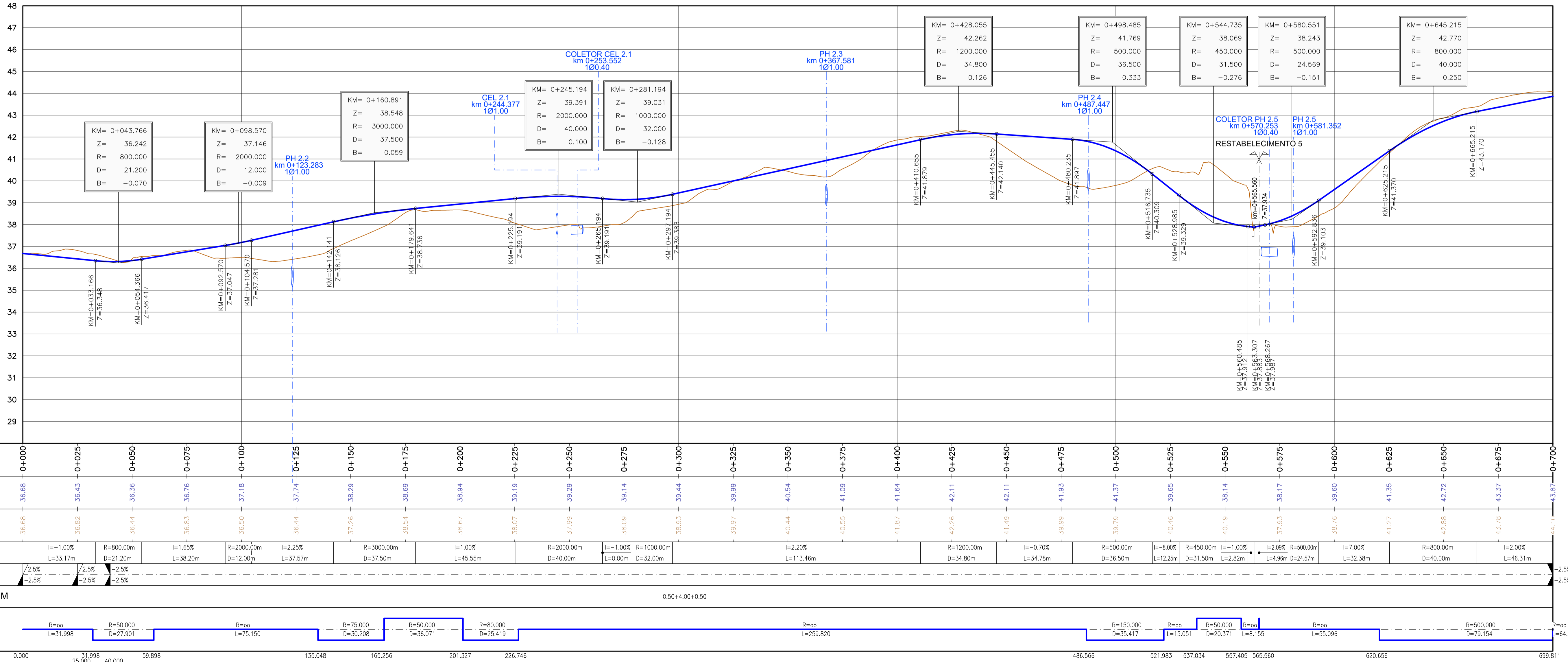
EN125 - VARIANTE DE OLHÃO RESTABELECIMENTO 4 (1/2) PERFIL LONGITUDINAL Esc. H=1:1000 V=1:100
