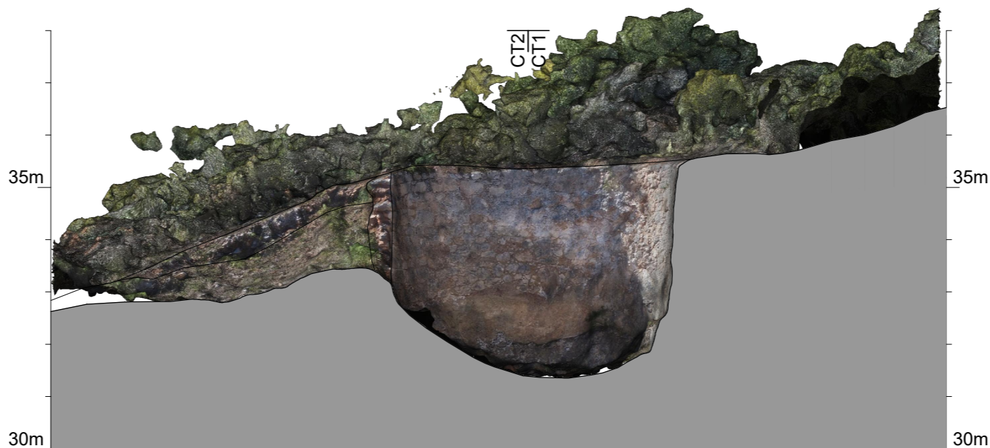
CORTE LONGITUDINAL 2
