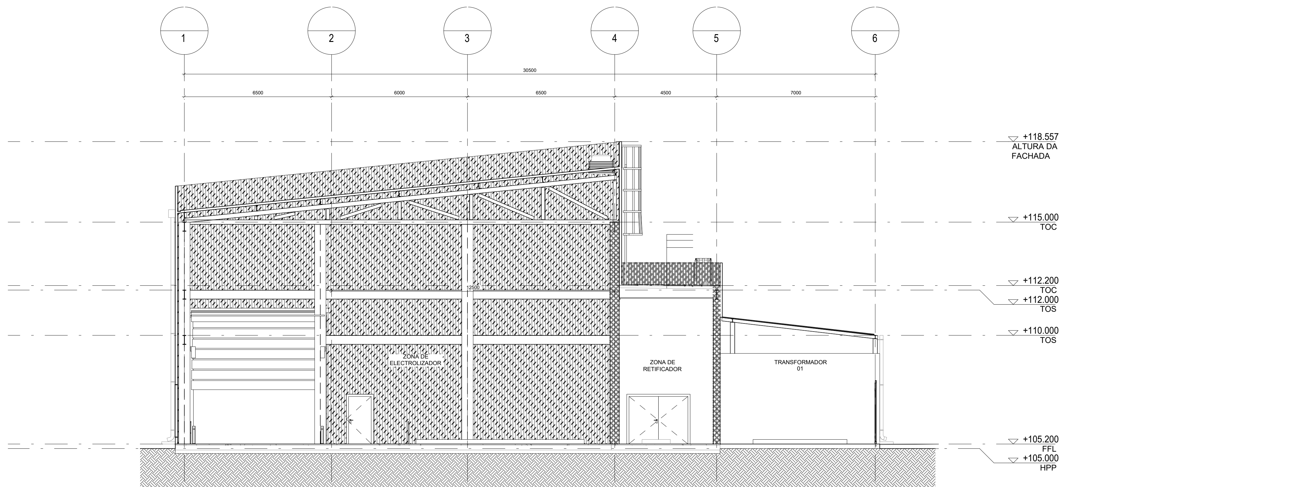
CORTE 2
