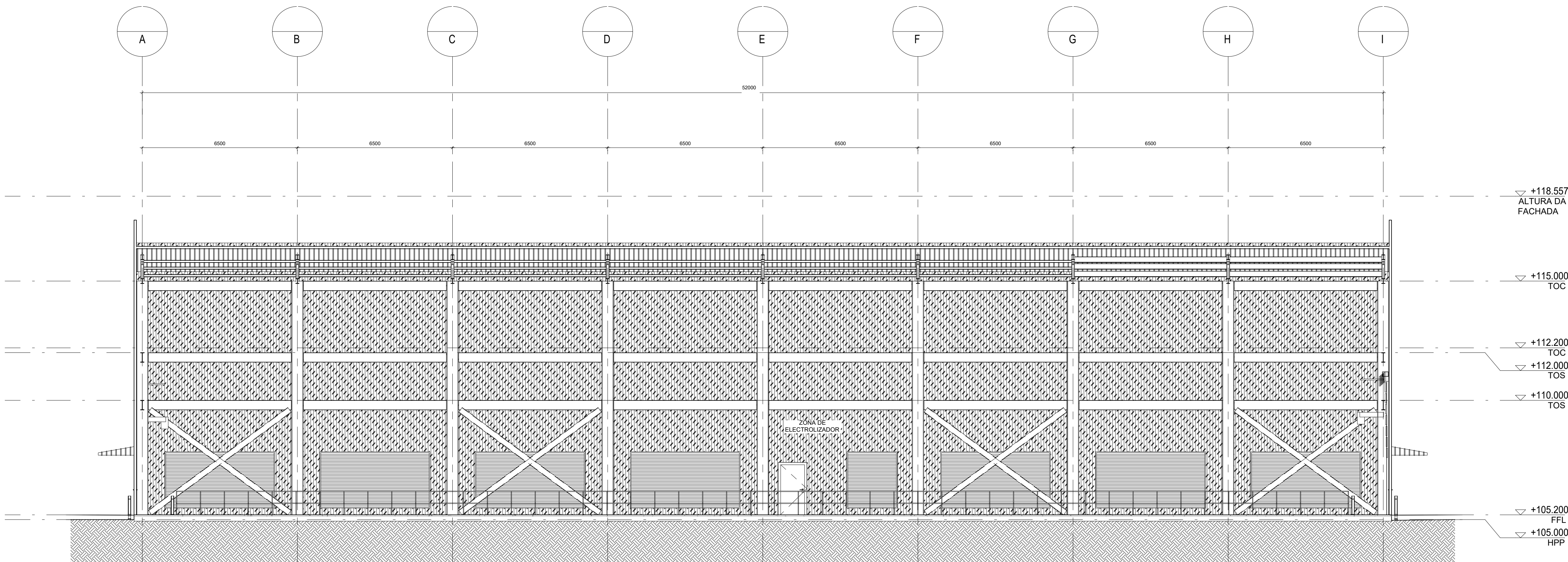
CORTE 1
