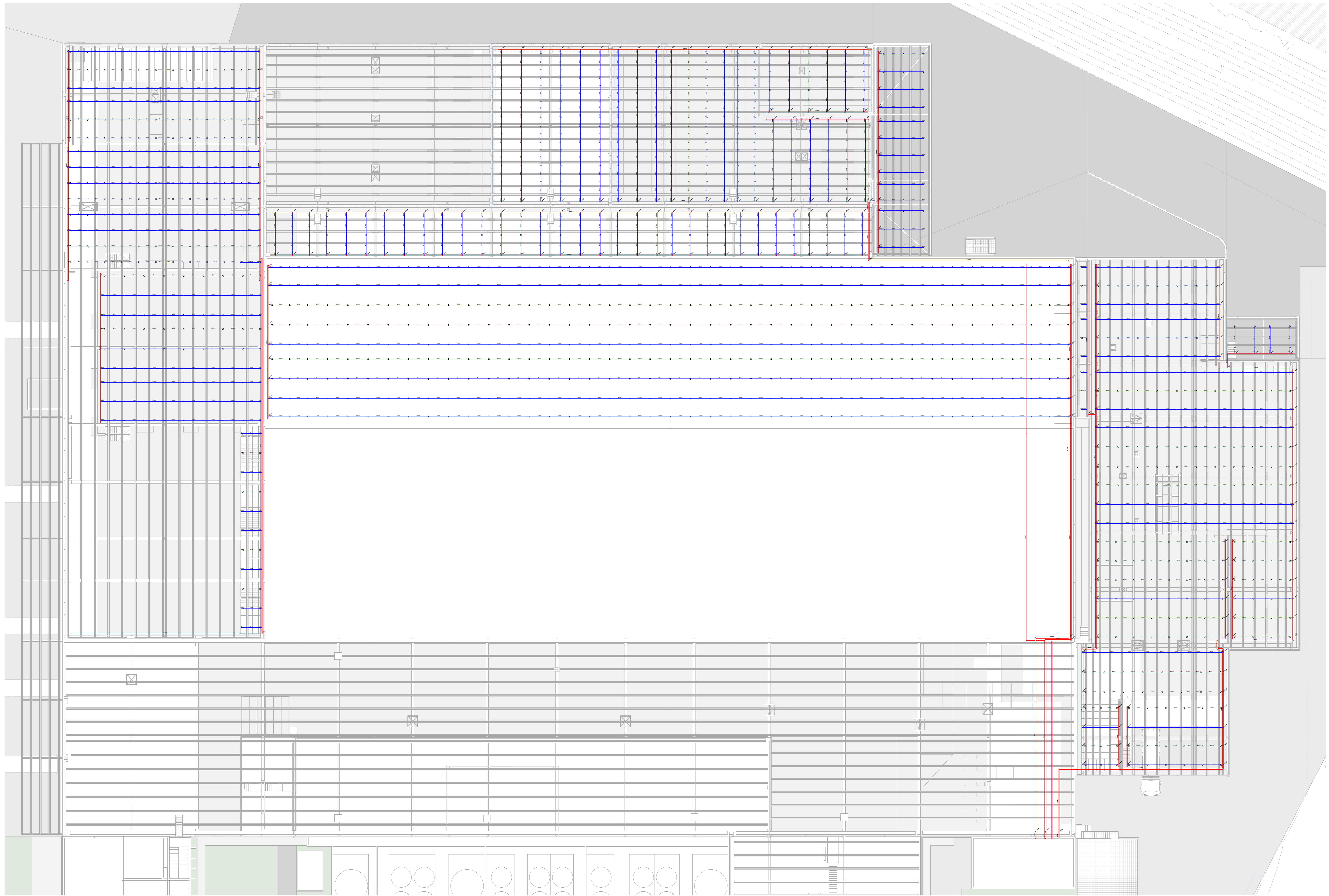
Cobertura Esc. 1:200
