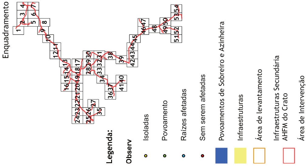
4.Planta da área de Povoamento de Sobreiro e Azinheira (9 de 9)
