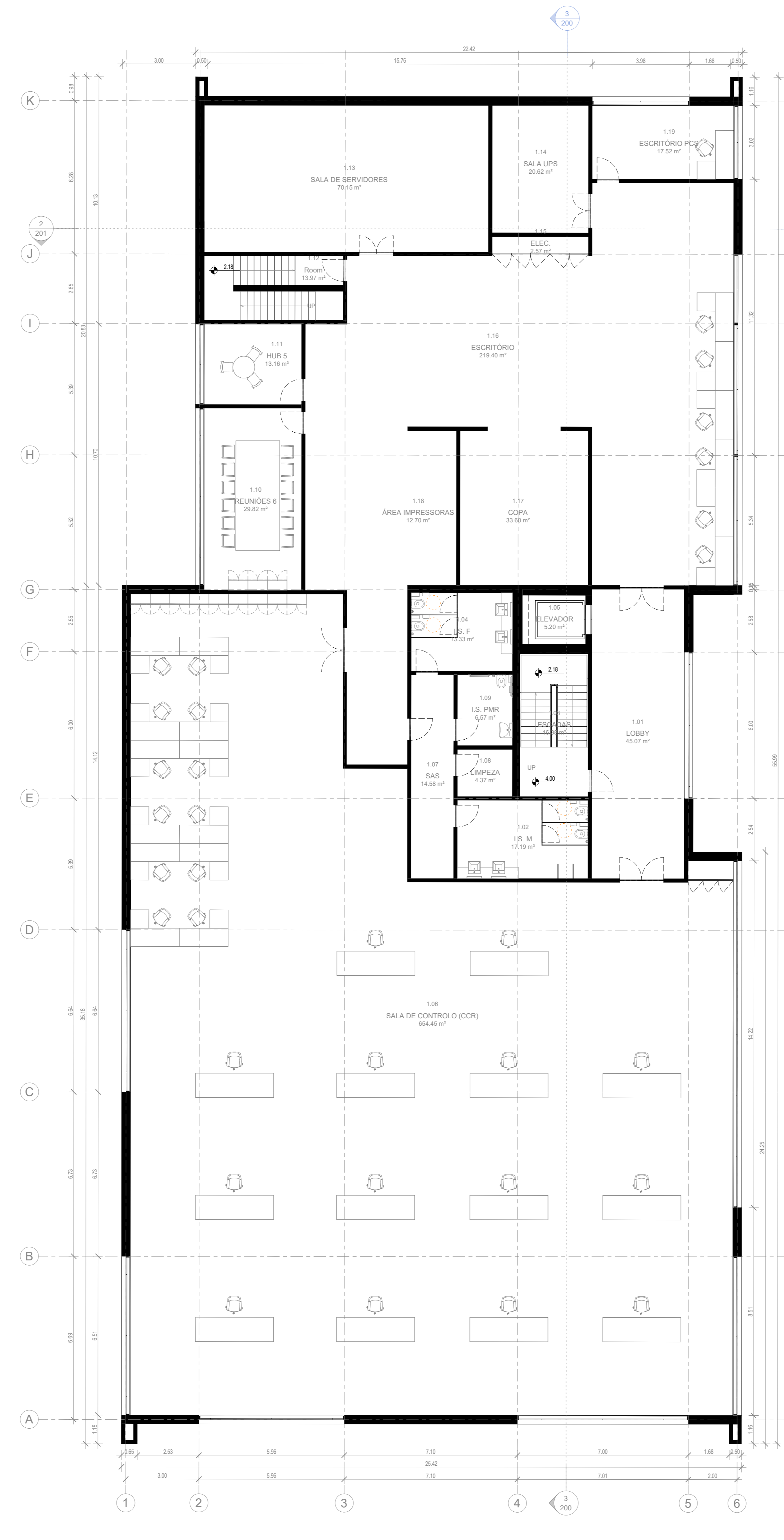
PLANTA - NÍVEL 01 1 : 100
