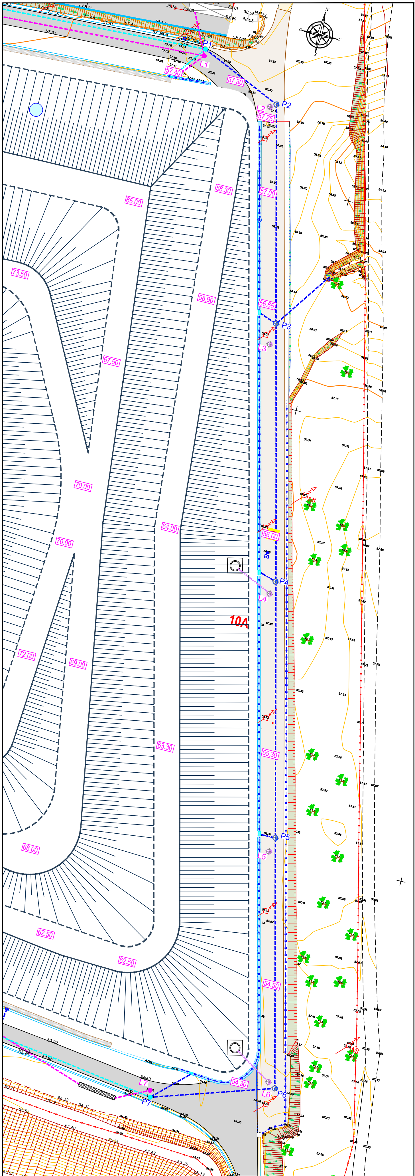
PLANTA DE LOCALIZAÇÃO DOS COLECTORES ESCALA: 1:500
