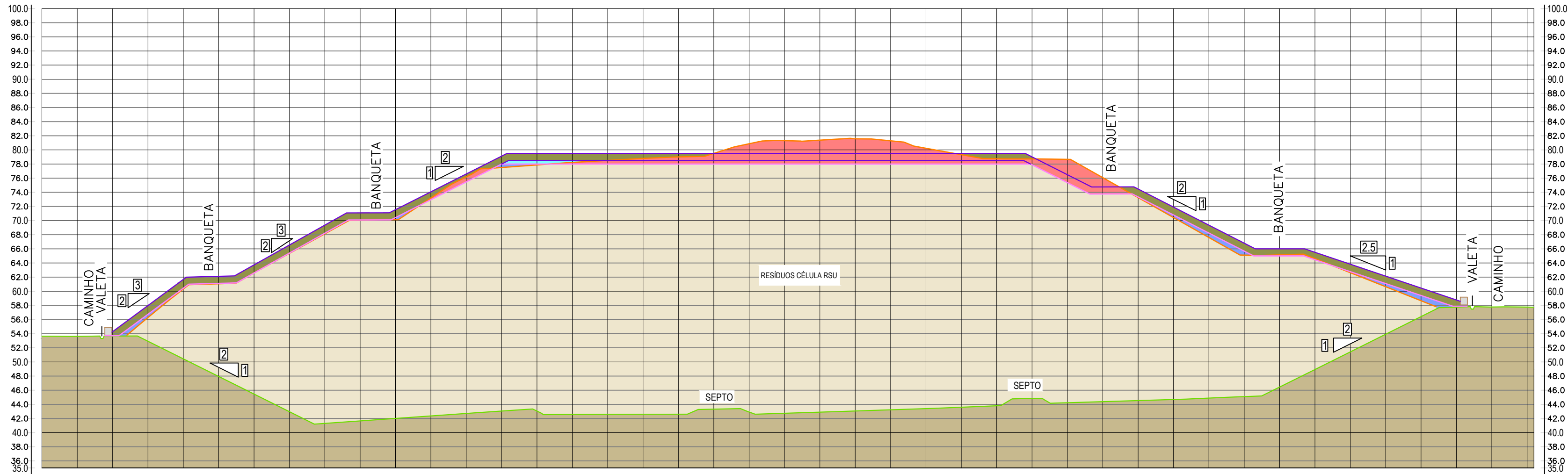
PERFIL LONGITUDINAL: PERFIL - 4 ESCALA HV: 500/500 DATUM: 35.00
