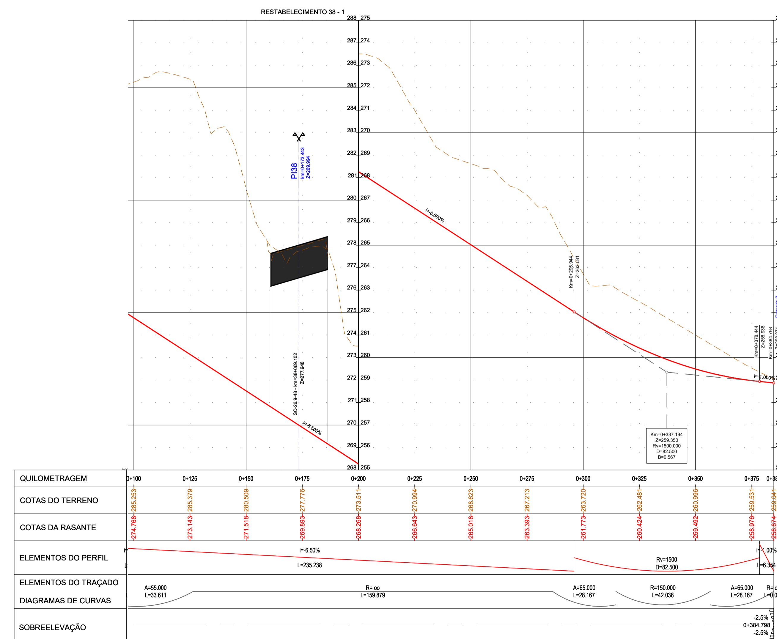
PERFIL LONGITUDINAL RESTABELECIMENTO 38-1 ESC. H= 1:1000 V= 1:100
