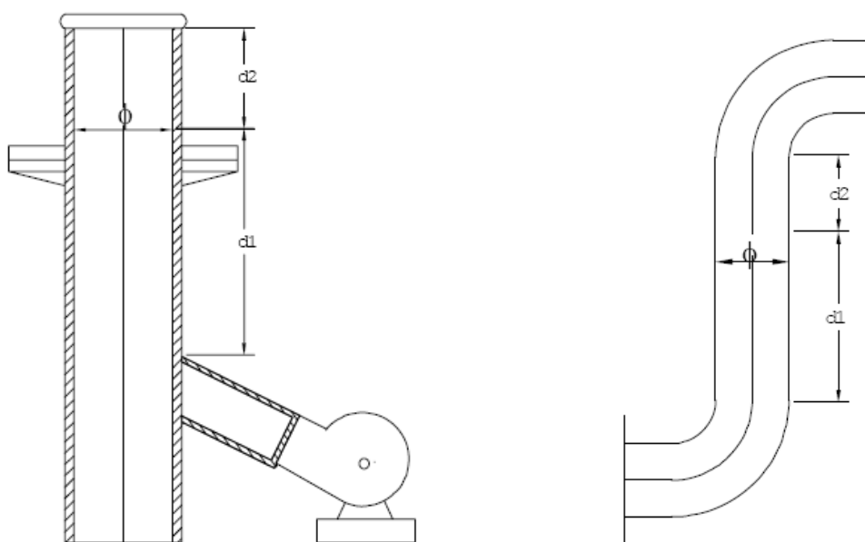
Figura 1 – Localização da secção de amostragem ( d_1 – distância a montante da toma de amostragem; d_2 – distância a jusante da toma de amostragem)
