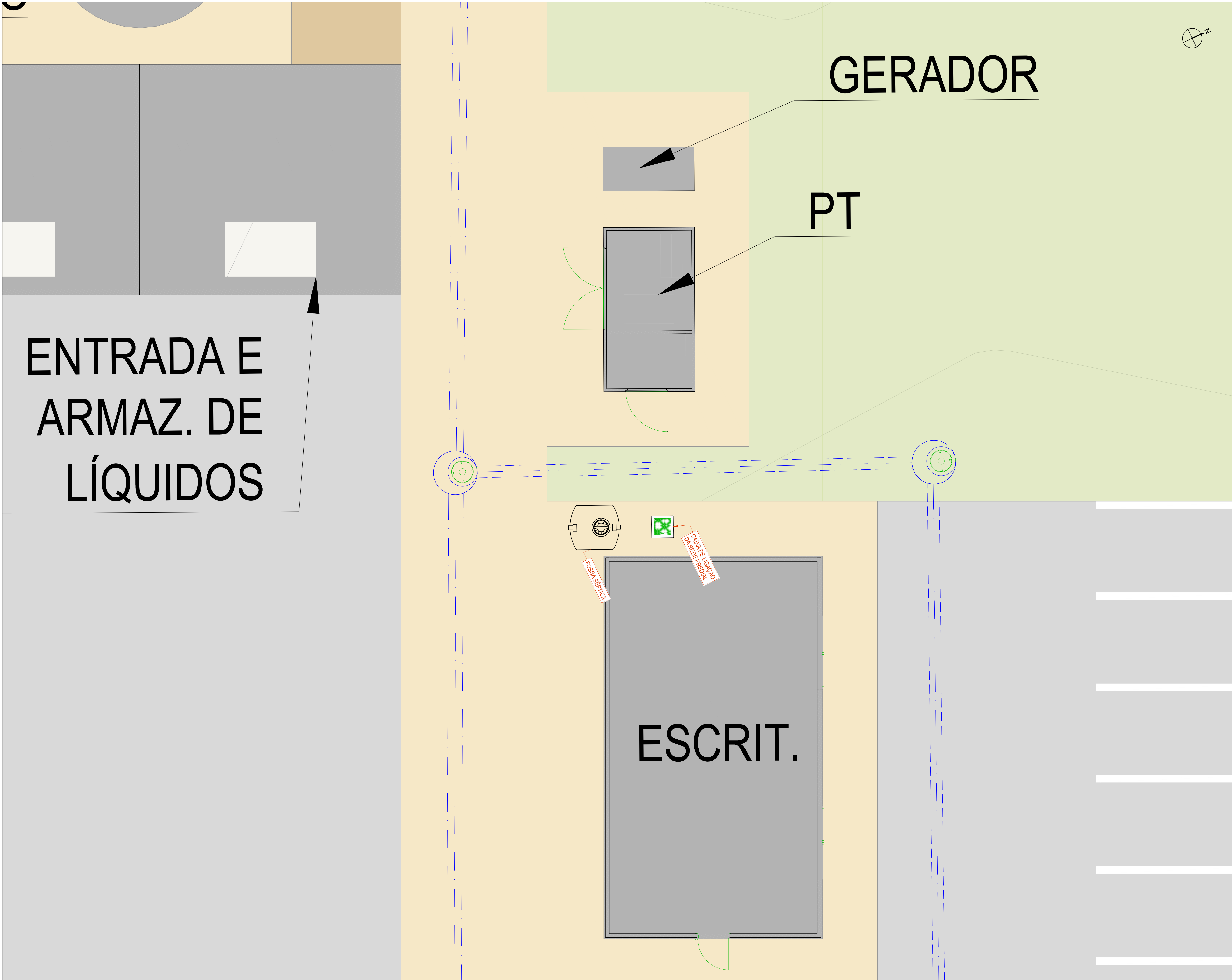
PLANTA ESCALA 1:500
