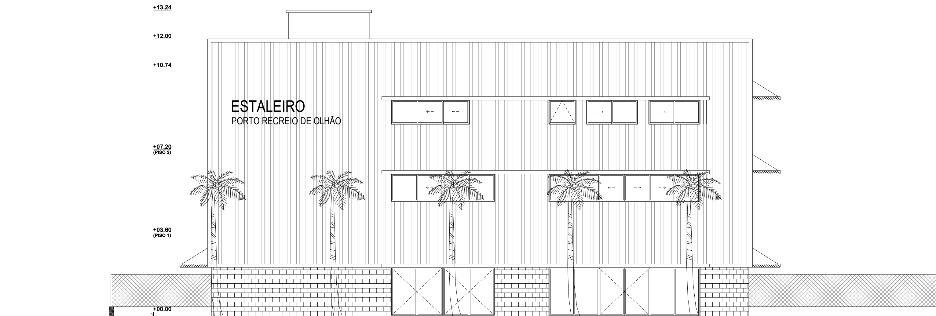
ALÇADO POENTE ESC. 1/100
