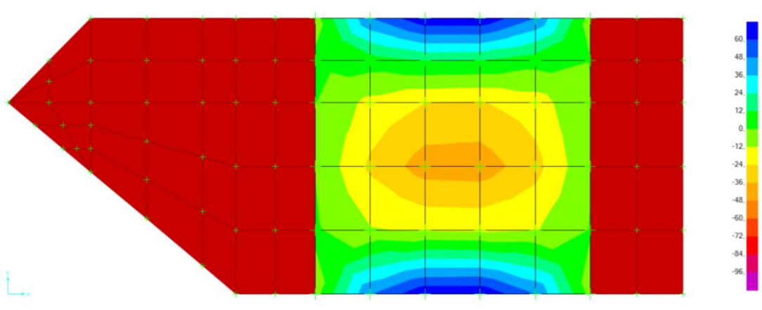
Figura 12.8 – Laje de fundo. Diagrama de Momentos Fletores Myy. Envoltente mínima
