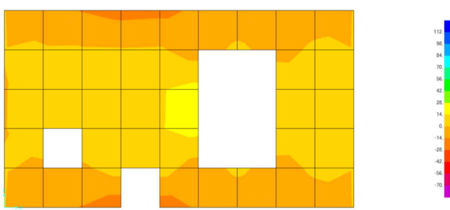
Figura 12.16 – Laje de topo. Diagrama de Momentos Fletores Myy. Envoltória máxima
