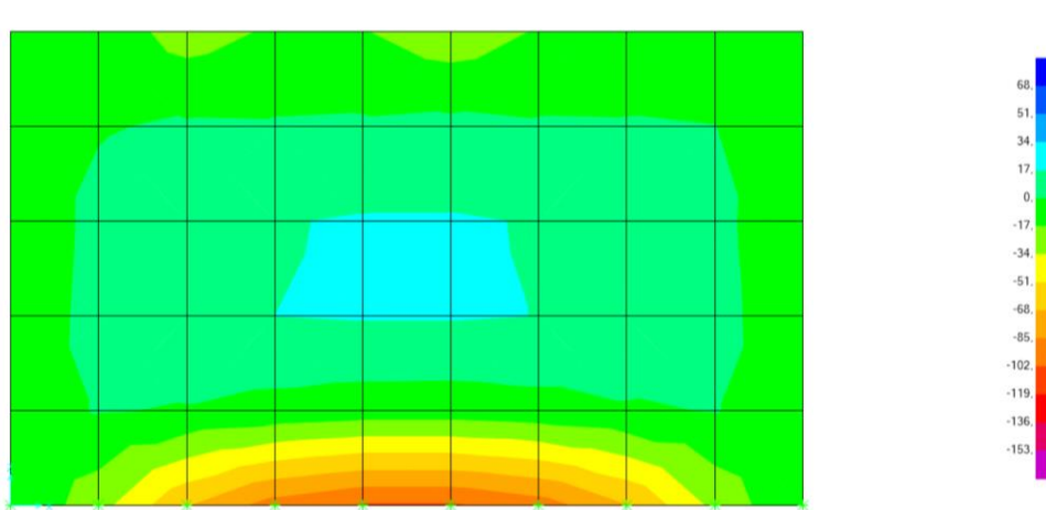
Figura 12.25 – Paredes. Diagrama de Momentos Fletores Myy. Envoltente mínima
