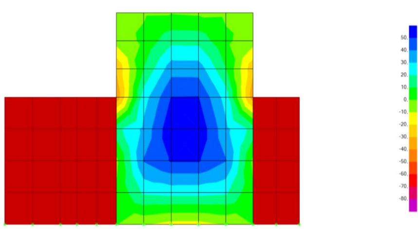
Figura 12.13 – Paredes. Diagrama de Momentos Fletores M_{xx} . Envolve máxima
