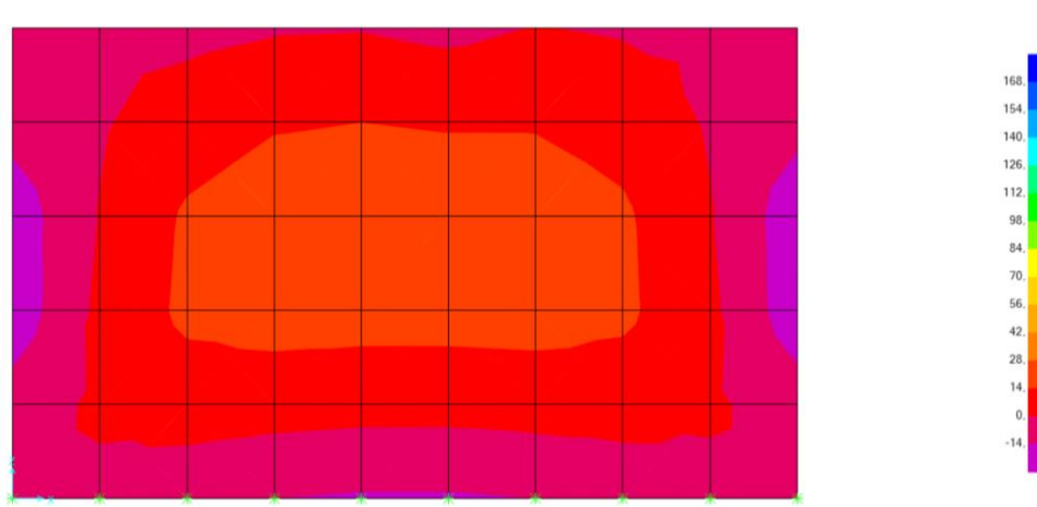
Figura 12.26 – Paredes. Diagrama de Momentos Fletores Mxx. Envoltente máxima
