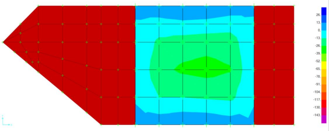
Figura 12.10 – Laje de fundo. Diagrama de Momentos Fletores Mxx. Envoltente mínima
