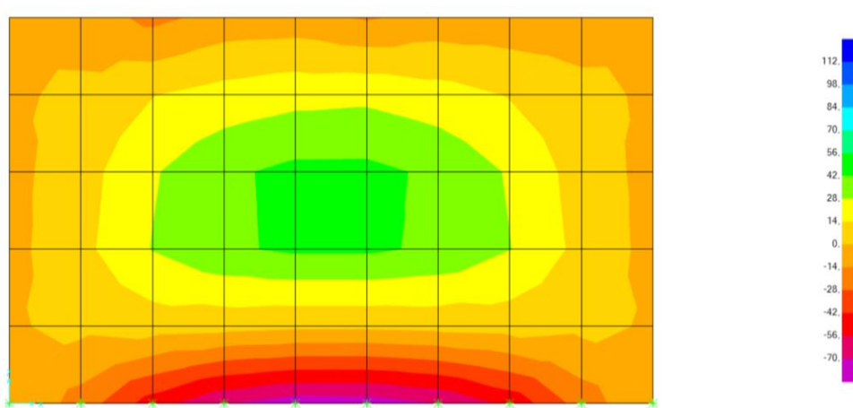
Figura 12.24 – Paredes. Diagrama de Momentos Fletores Myy. Envoltente máxima
