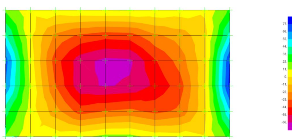
Figura 12.23 – Laje de fundo. Diagrama de Momentos Fletores Mxx. Envoltente mínima
