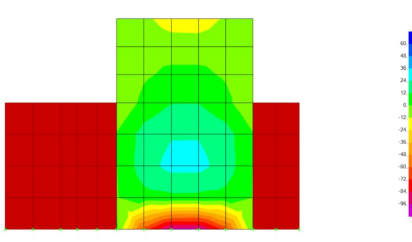
Figura 12.12 – Paredes. Diagrama de Momentos Fletores M_{yy} . Envolve mínima
