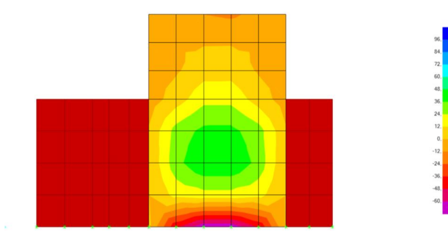
Figura 12.11 – Paredes. Diagrama de Momentos Fletores M_{yy} . Envolve máxima
