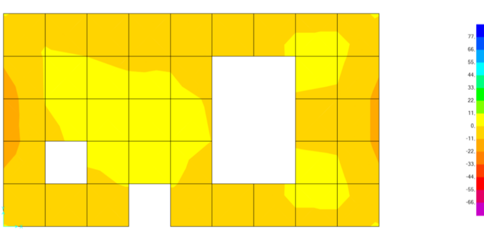
Figura 12.19 – Laje de topo. Diagrama de Momentos Fletores Mxx. Envolve mínima
