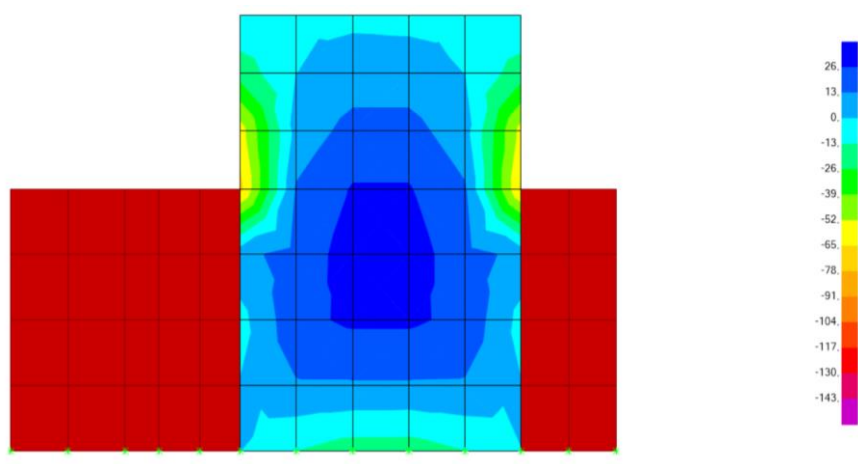
Figura 12.14 – Paredes. Diagrama de Momentos Fletores Mxx. Envoltória mínima
