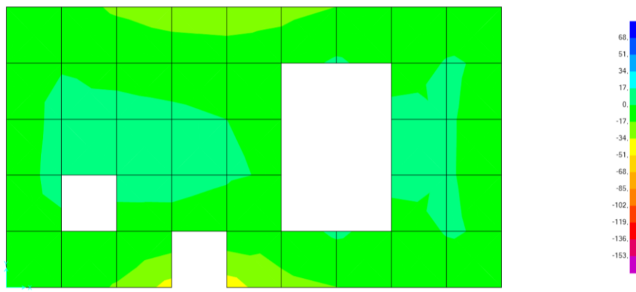
Figura 12.16 – Laje de topo. Diagrama de Momentos Fletores Myy. Envoltória máxima
