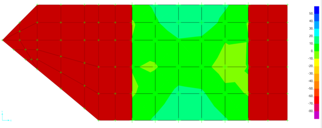
Figura 12.9 – Laje de fundo. Diagrama de Momentos Fletores Mxx. Envoltente máxima
