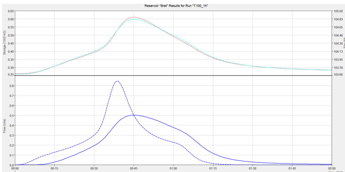
Figura 5.1 – Bacia de amortecimento e retenção - Gráfico de cima: Variação do volume acumulado no reservatório (linha vermelha) e da altura de água no seu interior (linha azul); em baixo: caudal afluyente (linha tracejada) e efluente (linha a cheio) do reservatório
