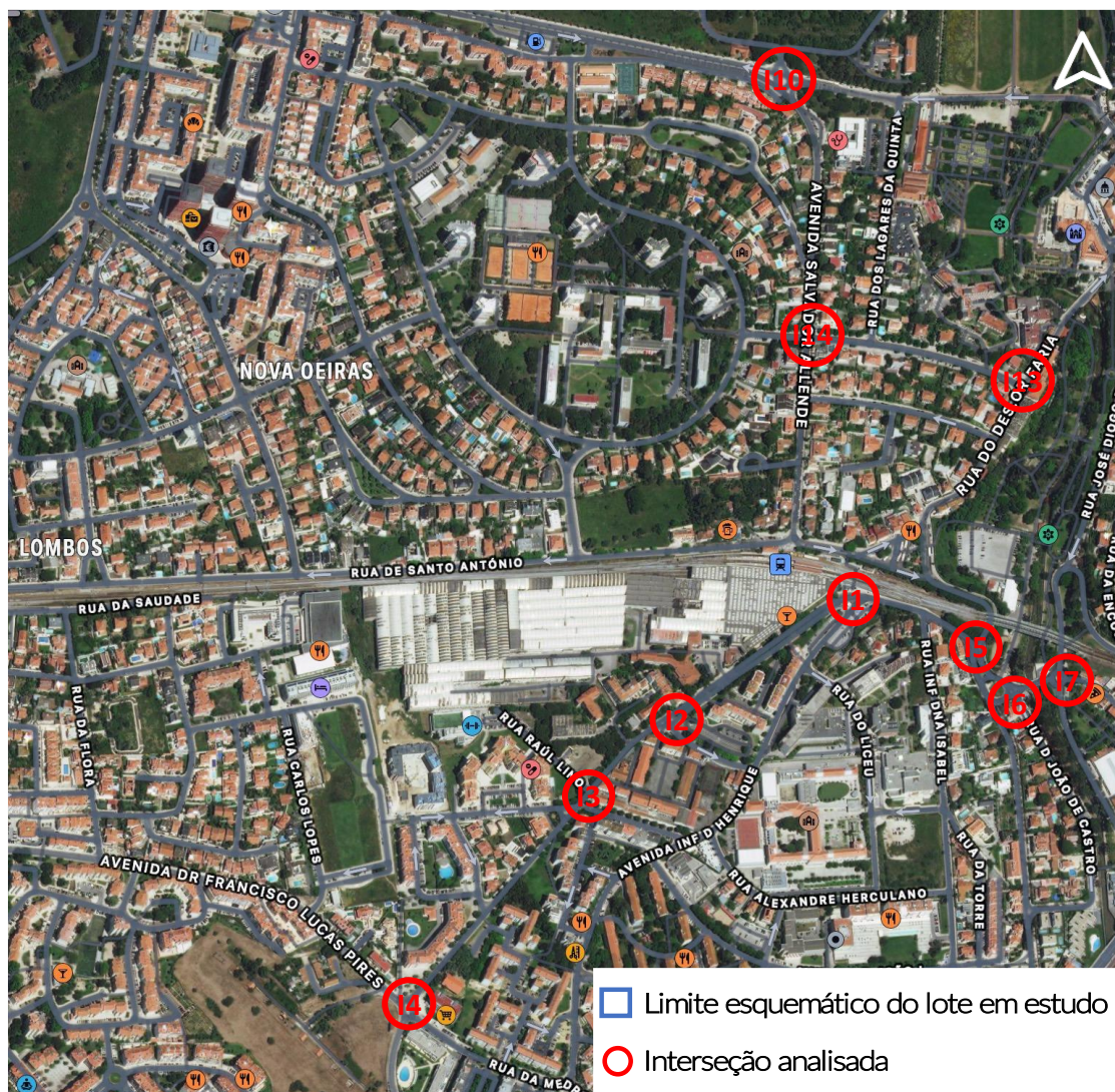
Figura 5.10.18 – Pontos singulares da rede rodoviária analisados no estudo de tráfego (FJ Consultores, 2022).
