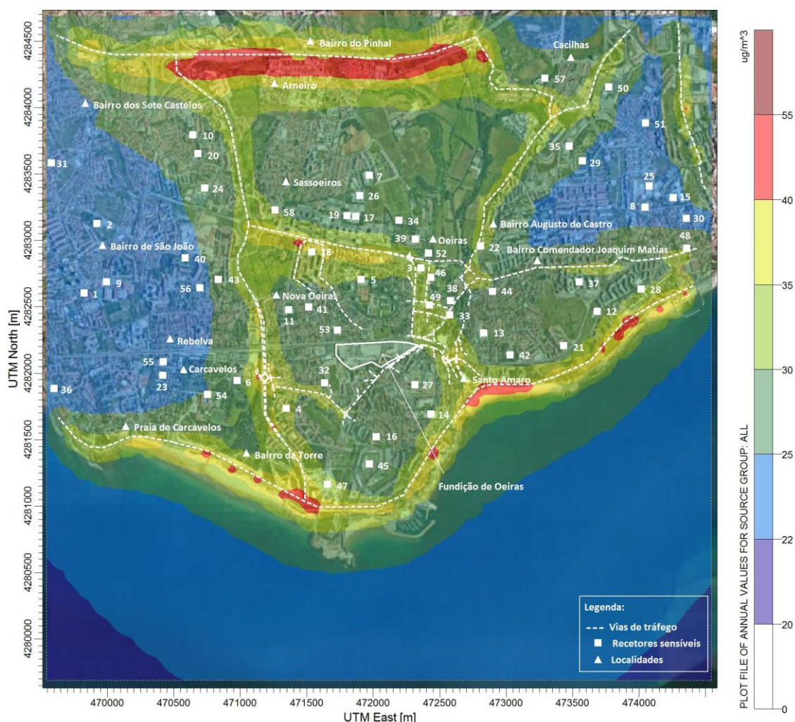
Figura 5.6.10 – Campo estimado das concentrações médias anuais de \text{NO}_2 ( \mu\text{g}\cdot\text{m}^{-3} ) verificadas no domínio em análise (situação atual).
