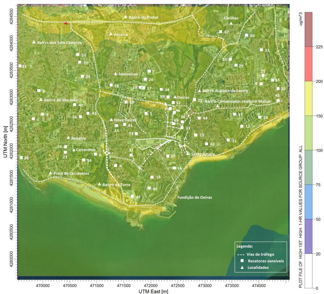
Figura 5.6.9 – Campo estimado das concentrações máximas das médias horárias de \text{NO}_2 ( \mu\text{g}\cdot\text{m}^{-3} ) verificadas no domínio em análise (situação atual).
