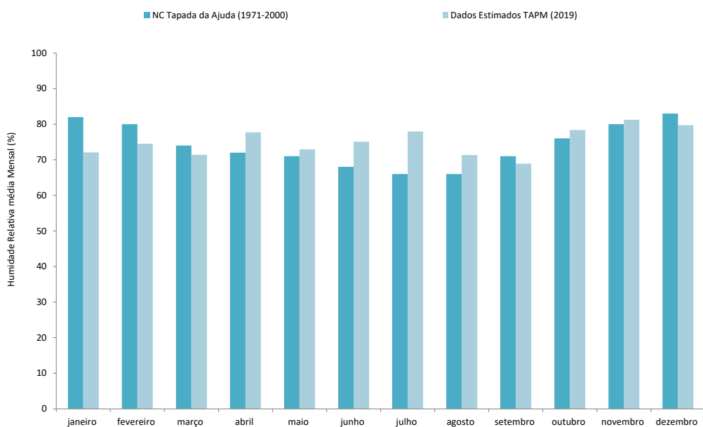
Figura 5.6.5 – Comparação das médias mensais de humidade relativa.
