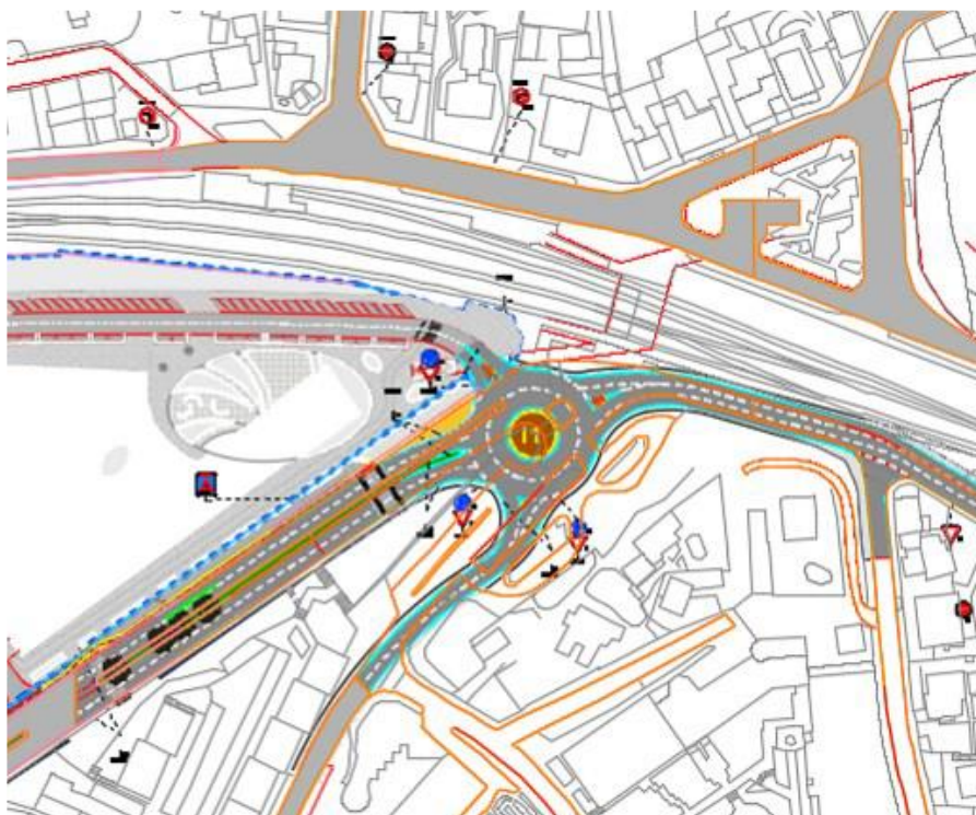
Figura 4.2.15 – Planta geral da rotunda I1.
