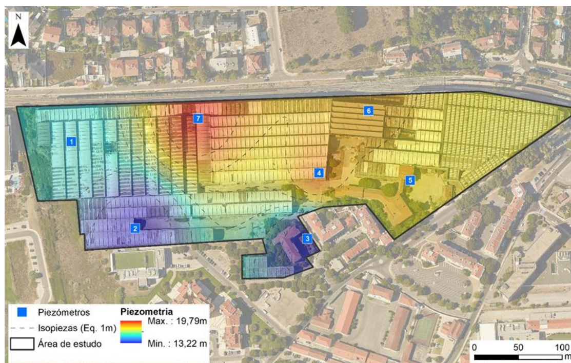
Figura 5.5.3 – Superfície piezométrica.
