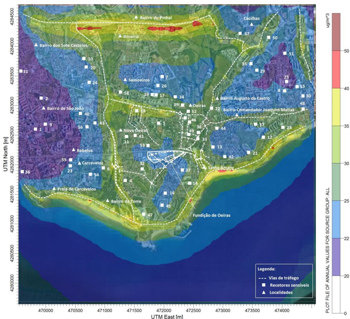
Figura 6.6.3 – Campo estimado das concentrações médias anuais de \text{NO}_2 ( \mu\text{g}\cdot\text{m}^{-3} ) verificadas no domínio em análise (situação futura).
