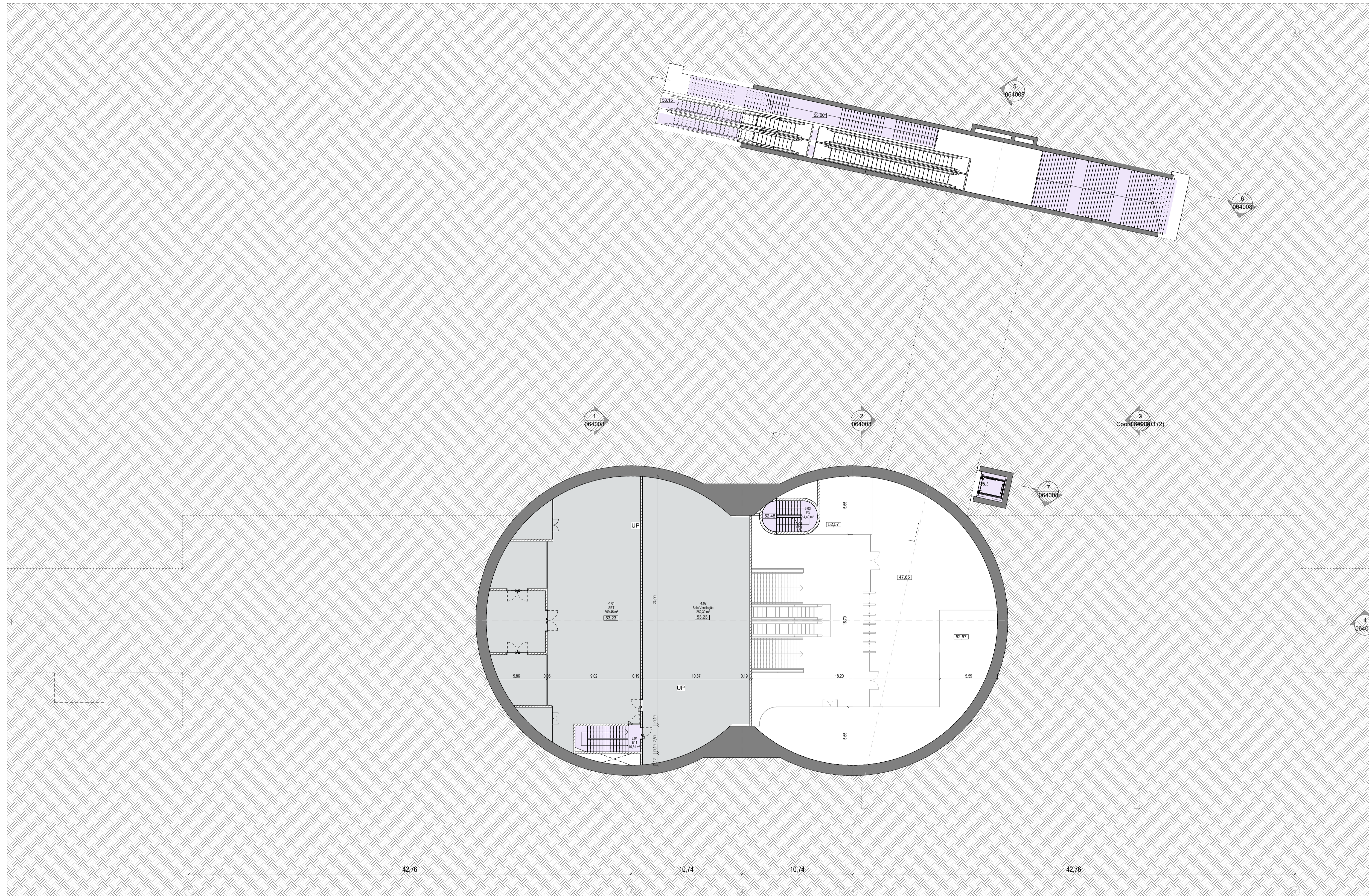
PLANTA DO SET E VENT 1 : 200
