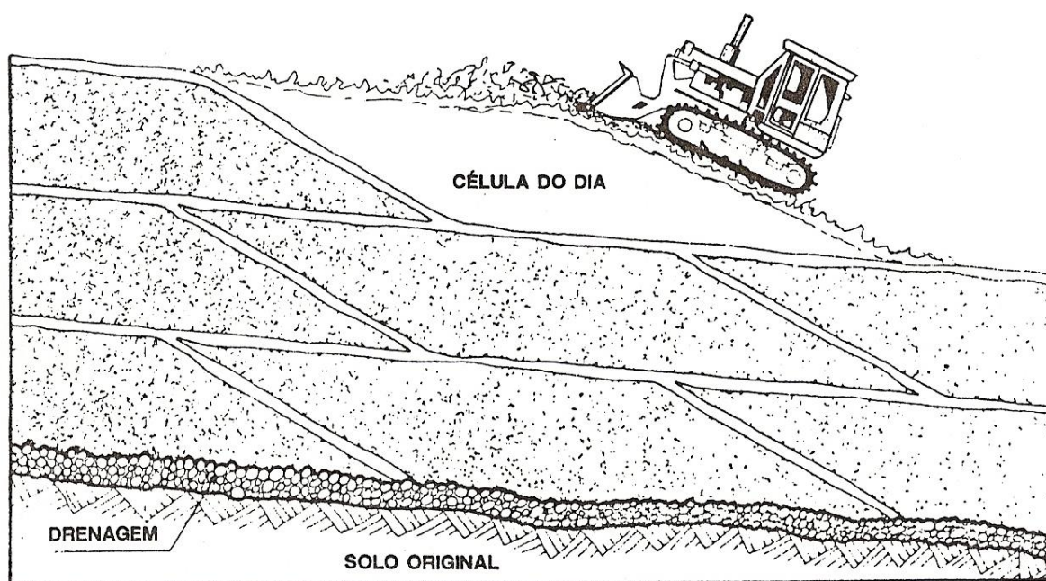
Figura 15 – Formação da Célula Diária.
