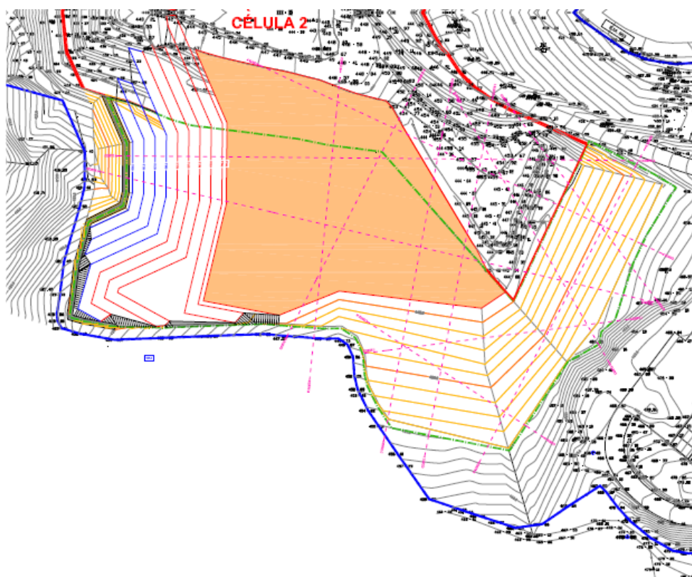
Figura 18 – Esquema de Enchimento Célula 3 – Fase 2.
