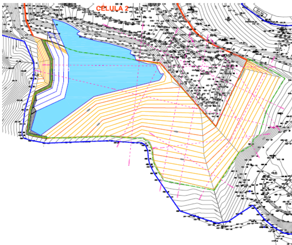
Figura 17 – Esquema de Enchimento Célula 3 – Fase 1.
