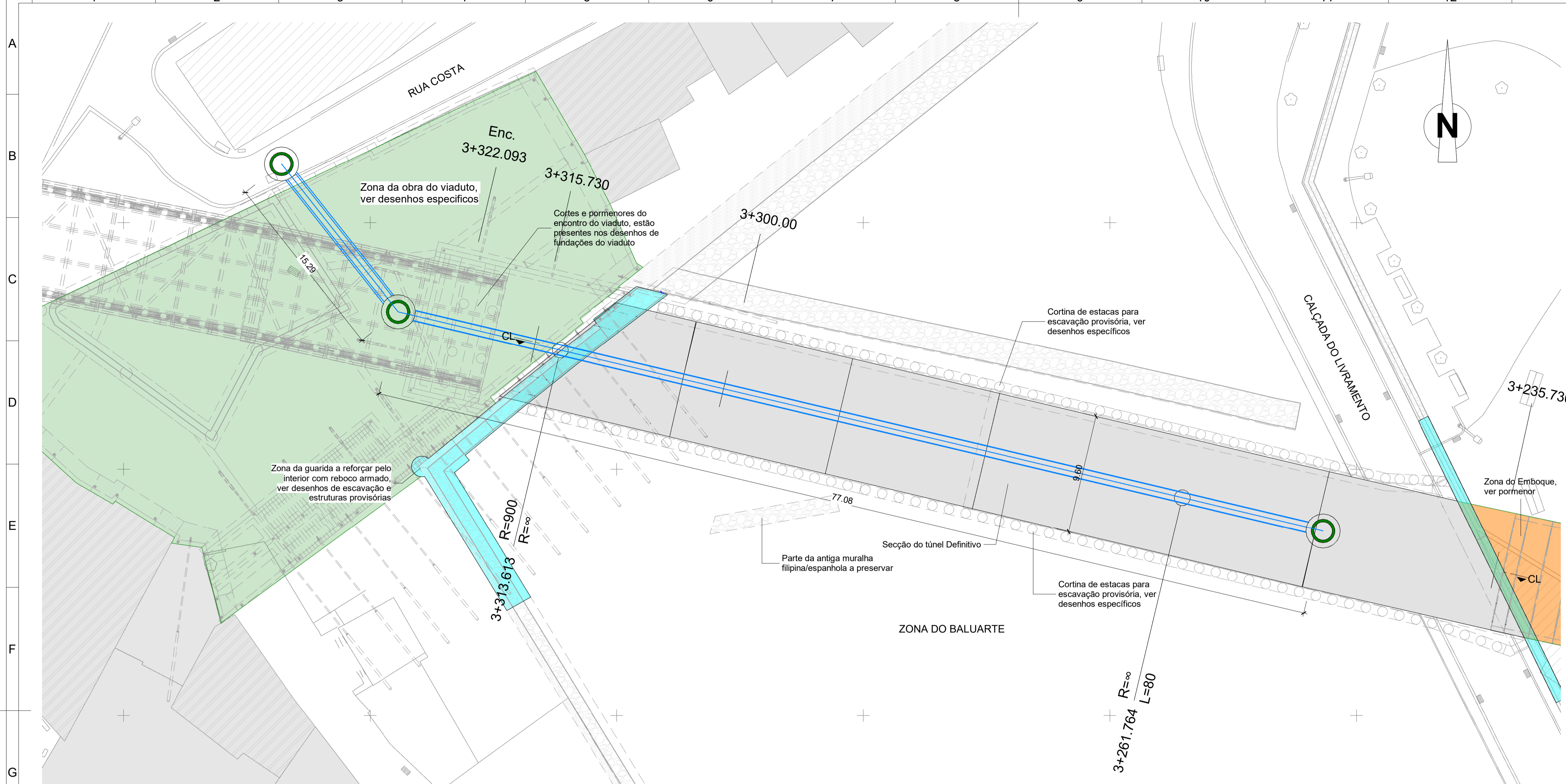
PLANTA DE DIMENSIONAMENTO Esc. 1 : 200
