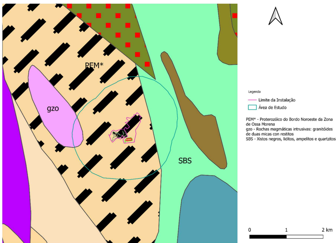
Figura 7.6 – Enquadramento geológico da área de estudo (adaptado de Camarate França et al (1963), Teixeira et al (1968), Zbyszewski et al (1965) e Zbyszewski et al (1974) ).
