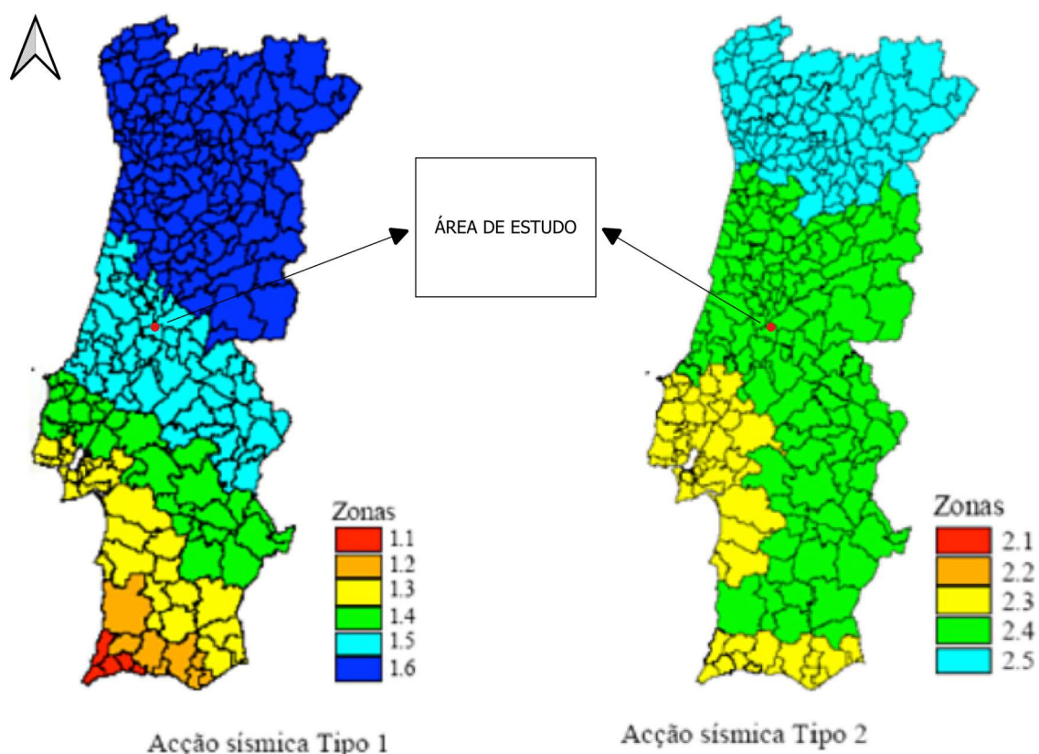
Figura 7.9- Zonamento sísmico na área de estudo definido no Anexo Nacional do Eurocódigo 8.
