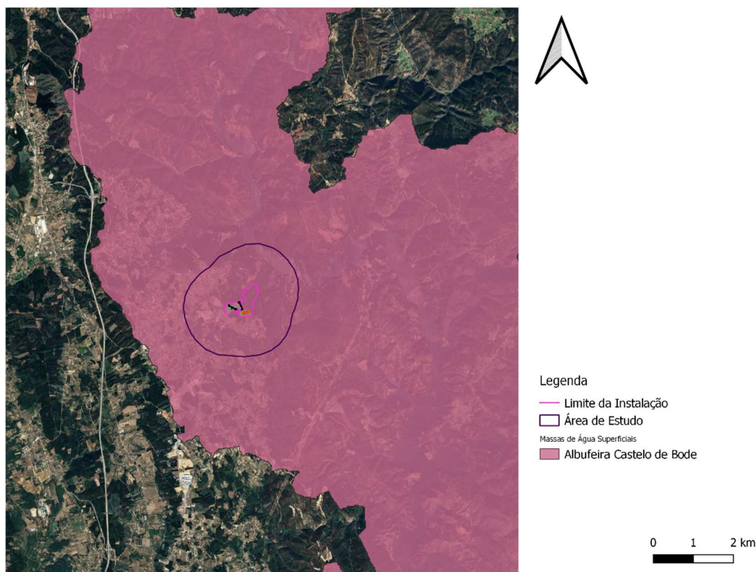
Figura 7.13 – Massas de Água Superficiais na área de estudo e envolvente
