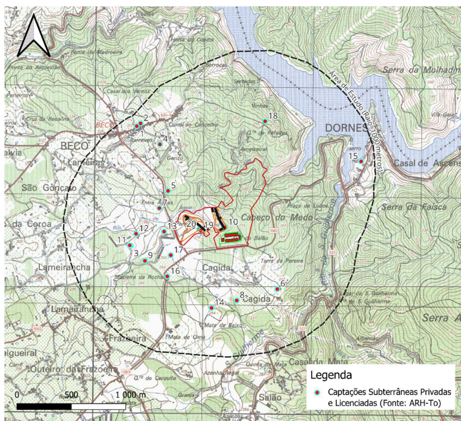
Figura 7.11 - Captações de água subterrânea privadas licenciadas na área em estudo, representadas sobre as Folhas 288 e 300 da Carta Militar de Portugal
