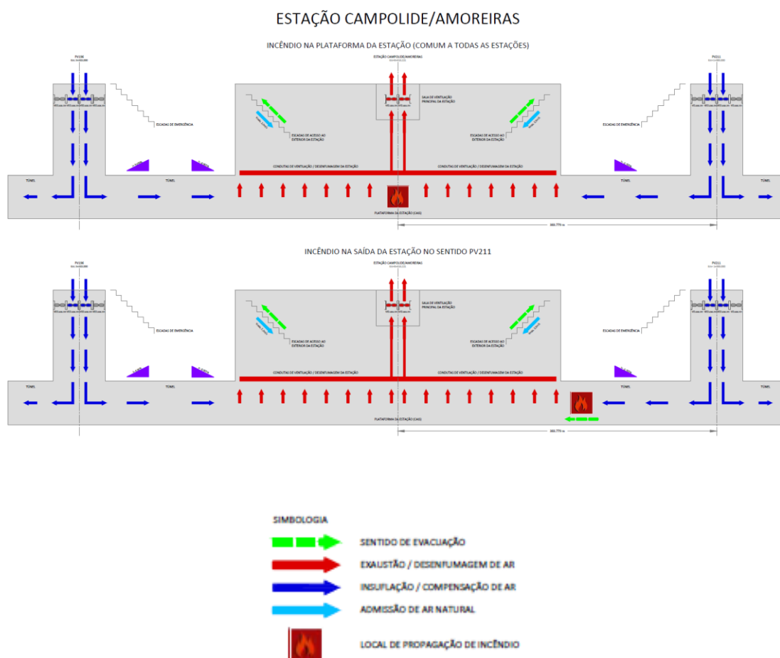
Figura 21 – Cenários de incêndio na estação Campolide/Amoreiras
