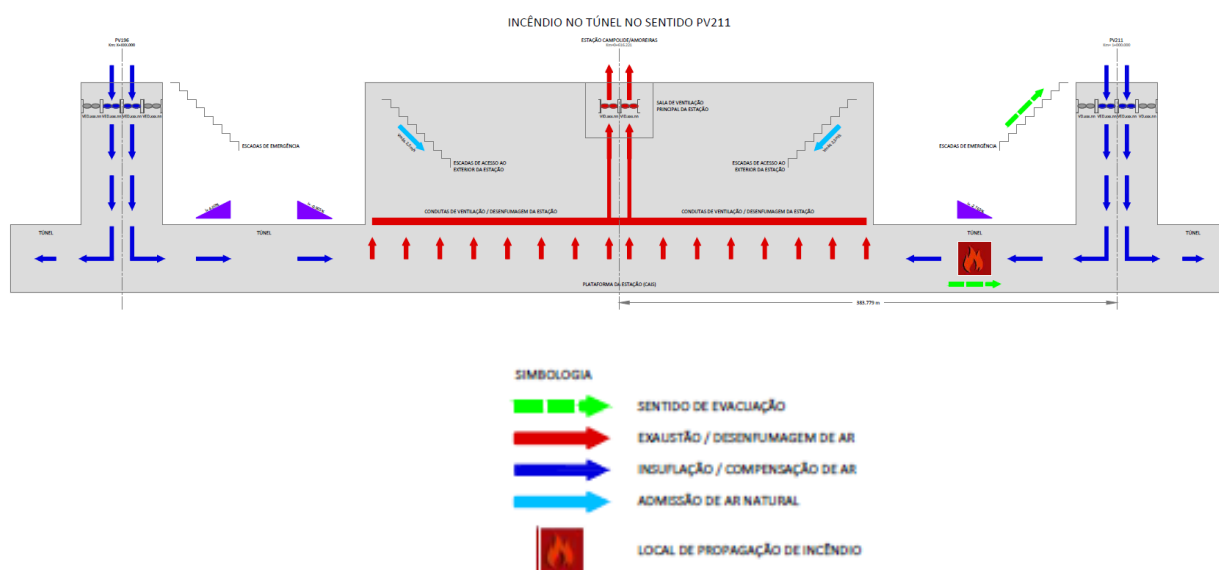
Figura 22 – Cenários de incêndio nos túneis adjacentes à estação
