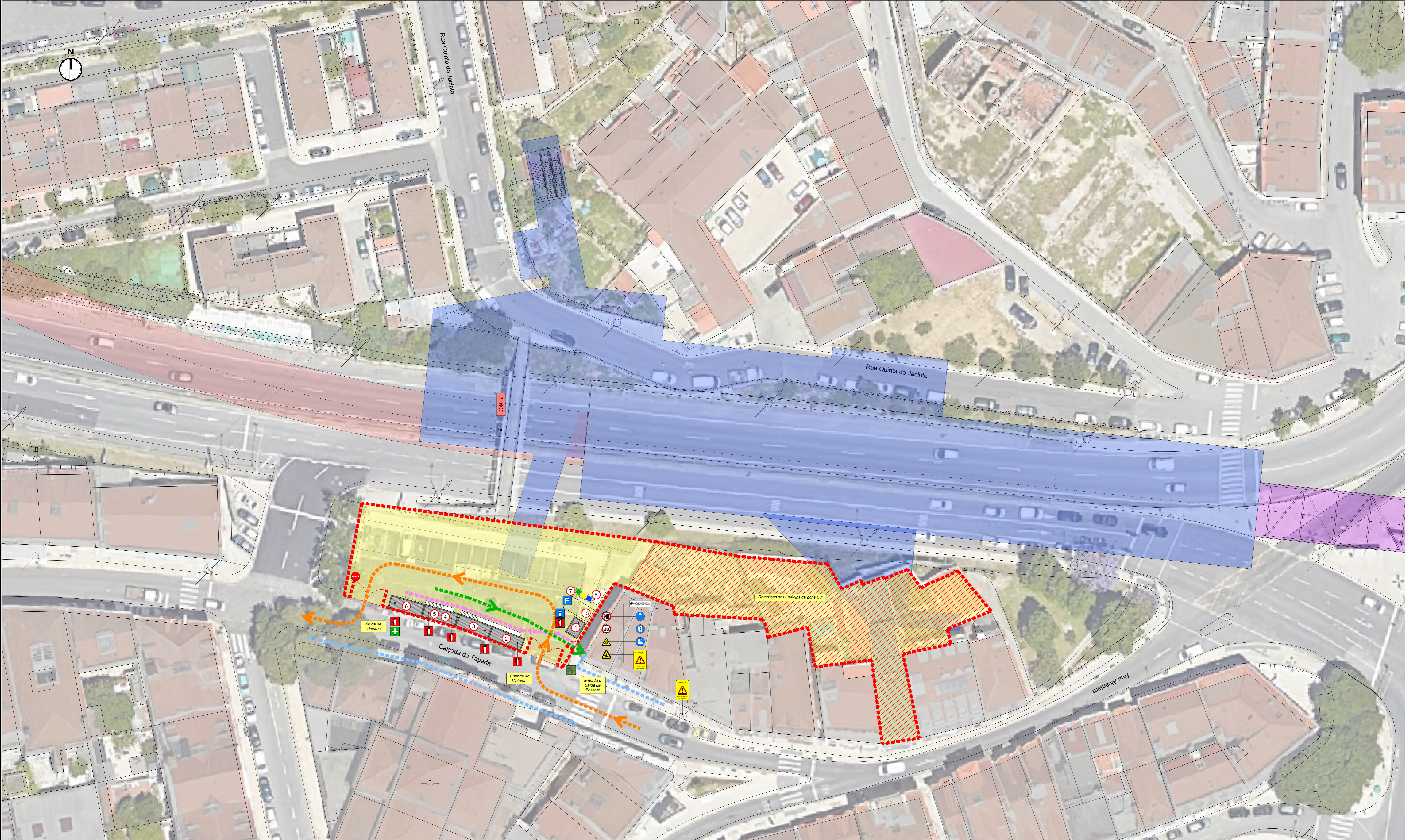
Estação Alcântara - Planta de Estaleiro e Sinalização de Segurança - Fase 1 A0 - Escala 1:250
