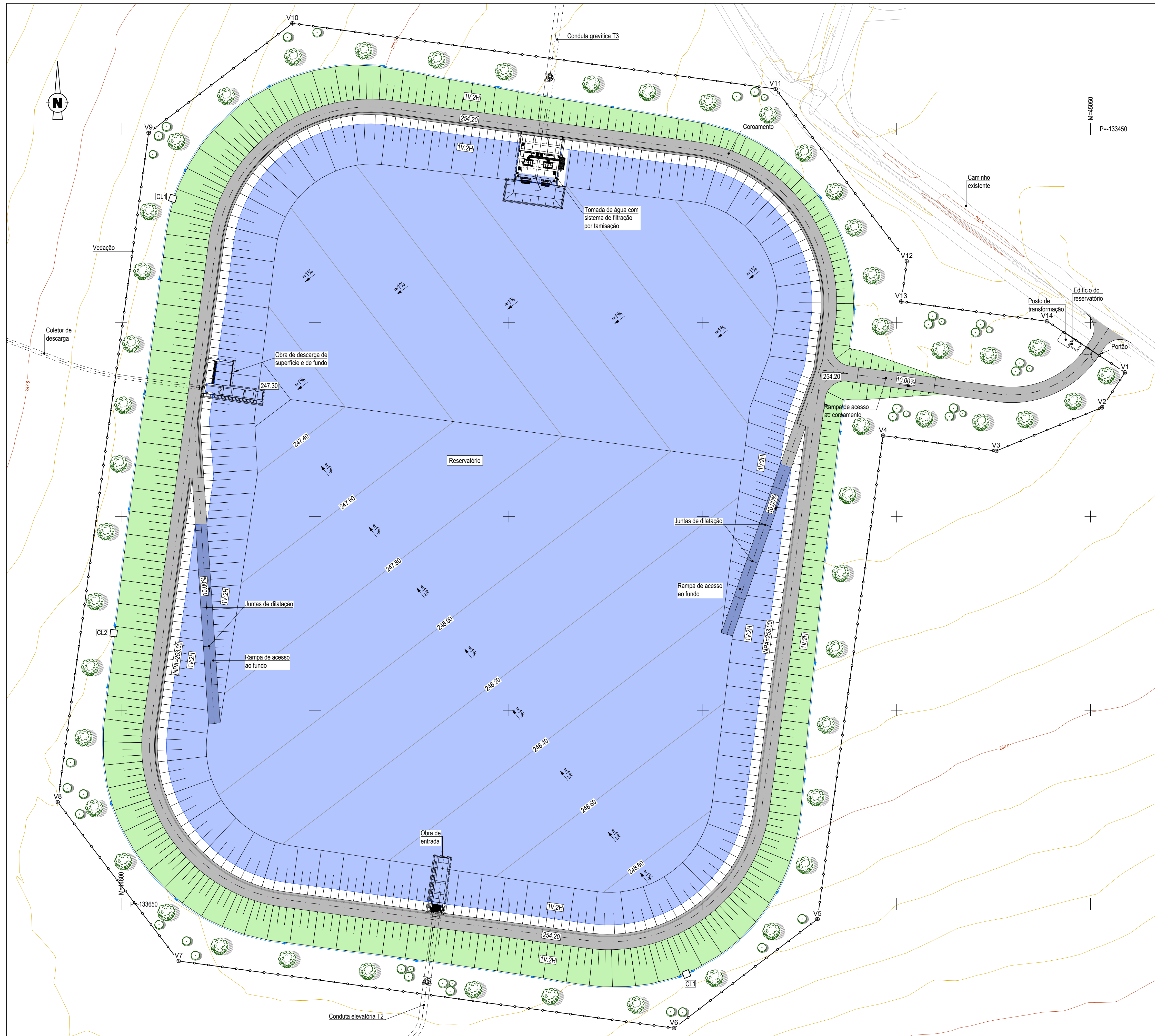
PLANTA Esc. 1:500
