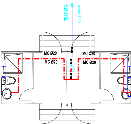
Planta Piso 1 - Edifício A
