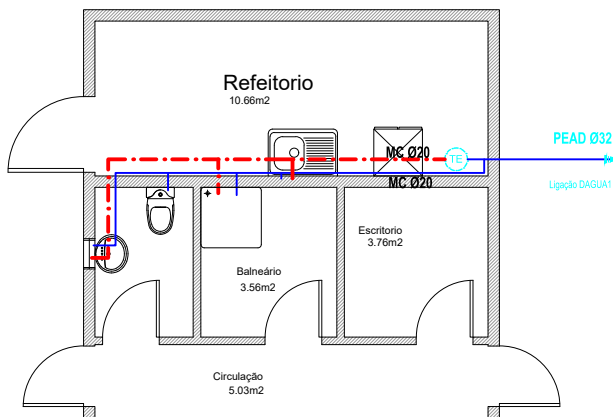
Planta Piso 1 - Edifício F
