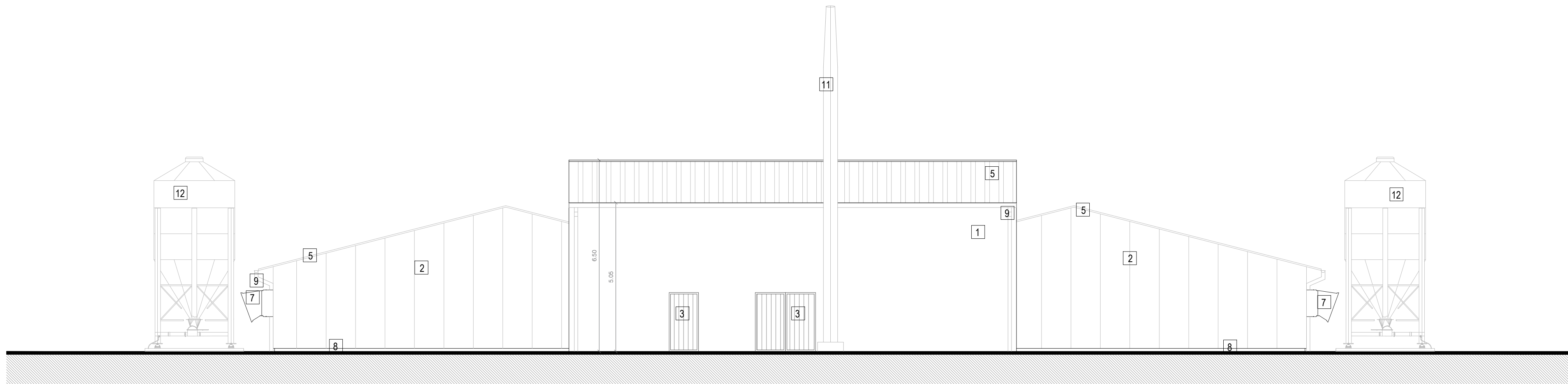
ALÇADO LATERAL ESQUERDO
