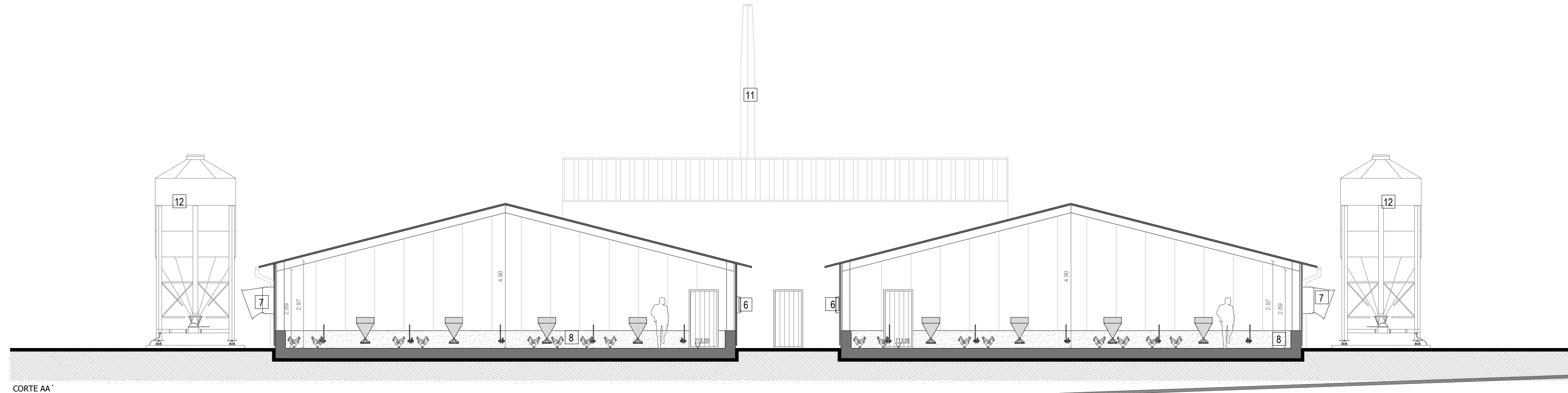
CORTE AA'
