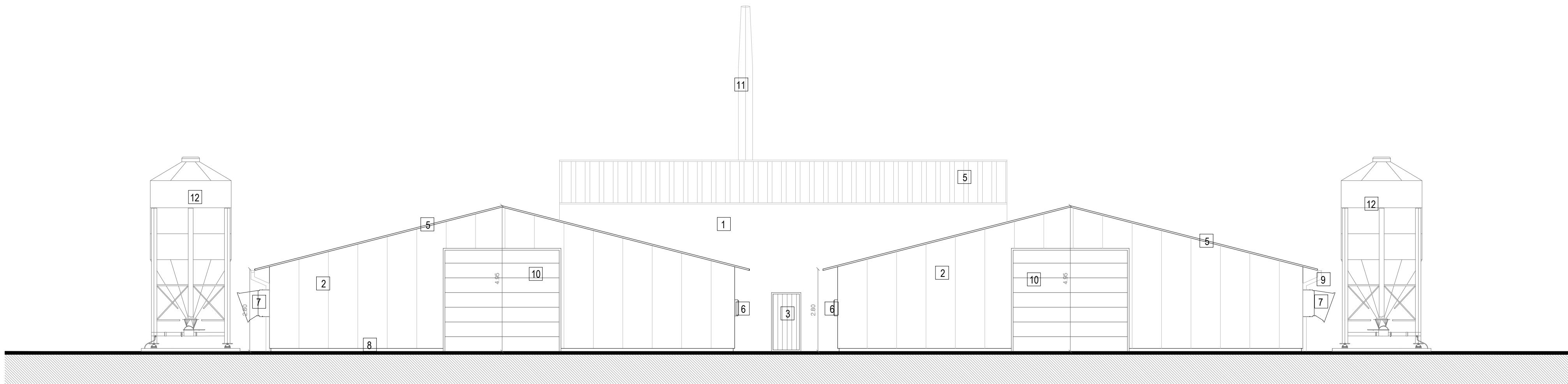
ALÇADO LATERAL DIREITO
