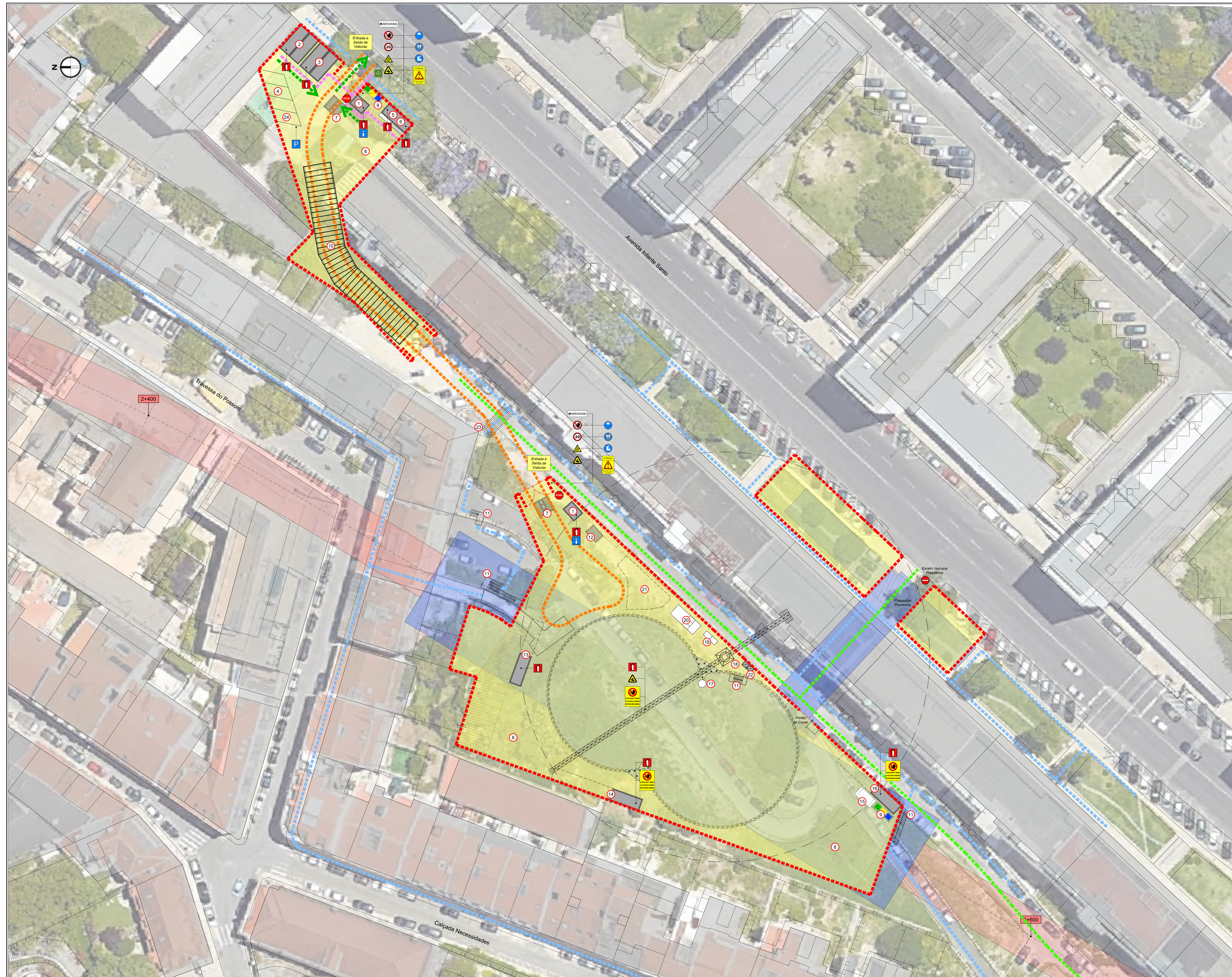
Estação Infante Santo - Planta de Estaleiro e Sinalização de Segurança A0 - Escala 1:250
