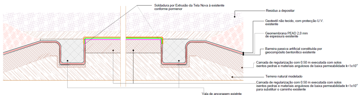
Figura 15 – Pormenor da ligação entre as células 1 e 2.
