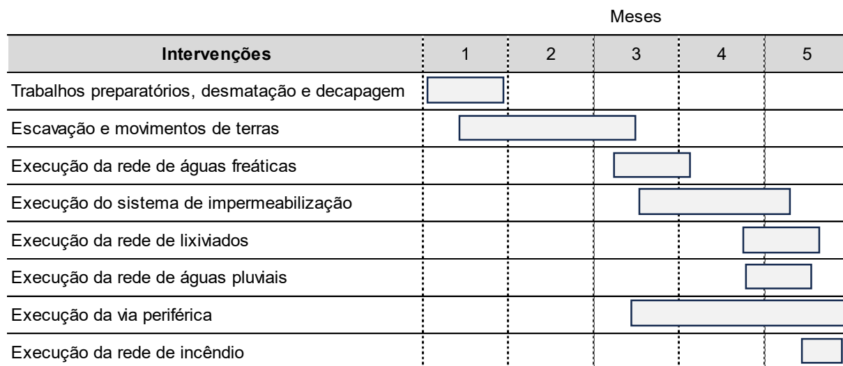
Figura 18 - Planificação da fase de construção.
