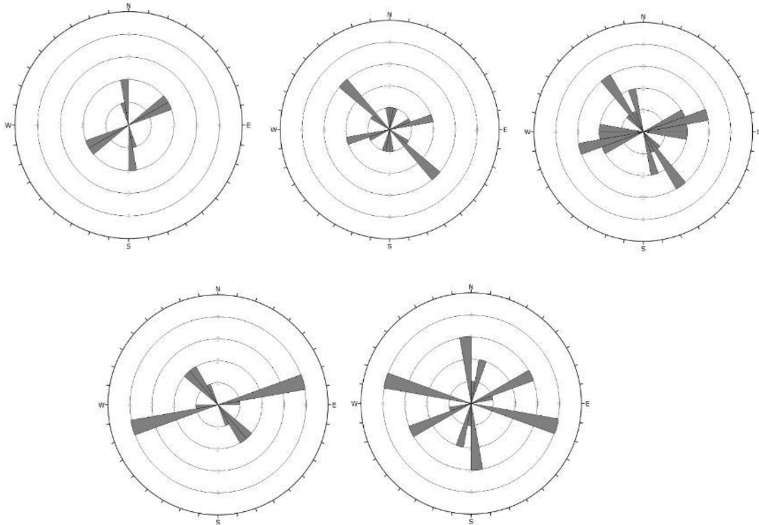
Figura 26 – Diagramas de Roseta representativos das principais famílias de diáclases em cada uma das estações geológicas (da esquerda para a direita – estações 1, 2, 3, em cima, e estações 4 e 5, em baixo).
