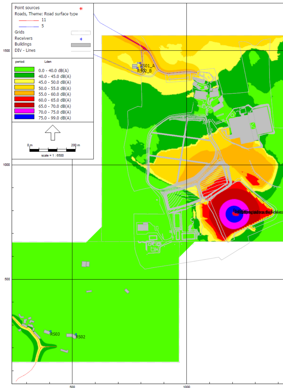
Figura 280 - Mapa de Ruído, calculado a 4 metros, indicador diurno-entardecer-noturno (Lden) – situação resultante – cenário 1.
