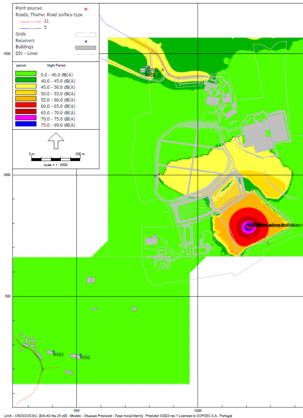
Figura 281 – Mapa de Ruído, calculado a 4 metros, indicador noturno (Ln) – situação resultante – cenário 1.
