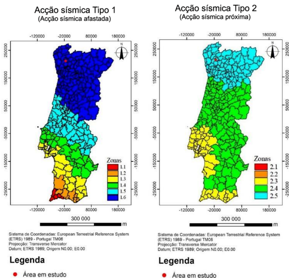
Figura 38 – Zonamento sísmico do Anexo Nacional da EN 1998-1 (EC8), com identificação da área em estudo.
