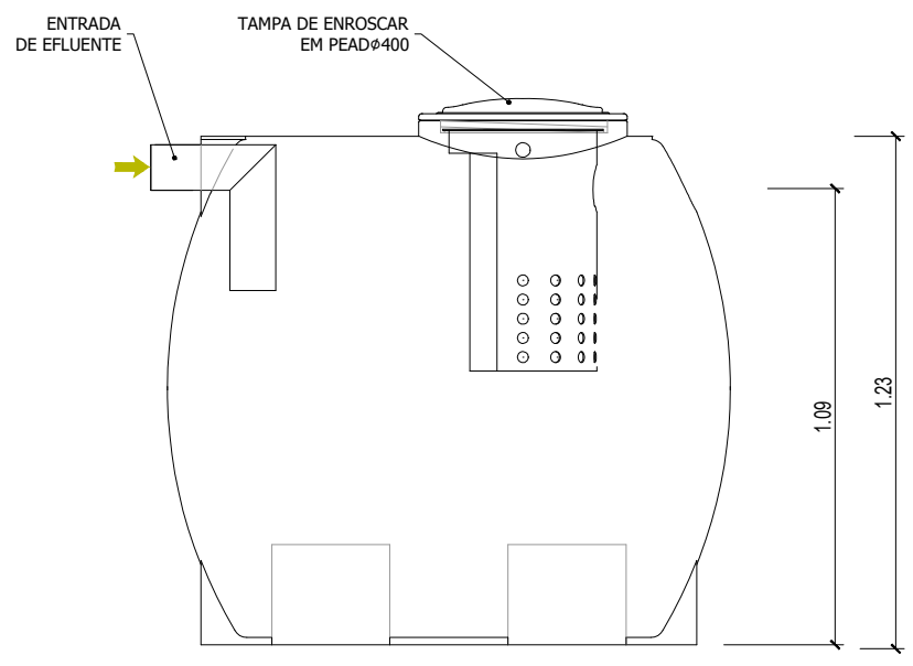
CORTE LONGITUDINAL DA FOSSA SÉPTICA ESCALA 1:20
