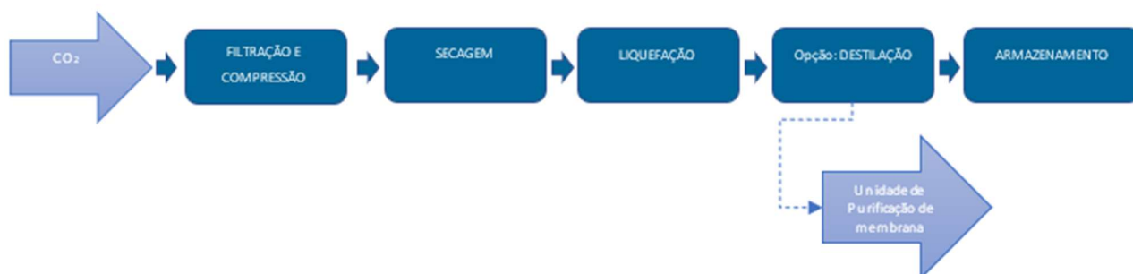
Figura 9 - Sistema de liquefação e armazenamento de CO 2 biogénico
