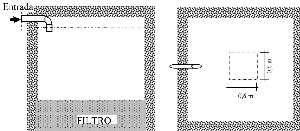
Figura 2 – Fossa séptica com poço absorvente
