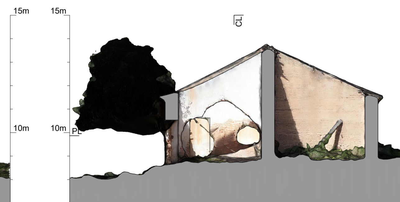
CORTE TRANSVERSAL (E53)
