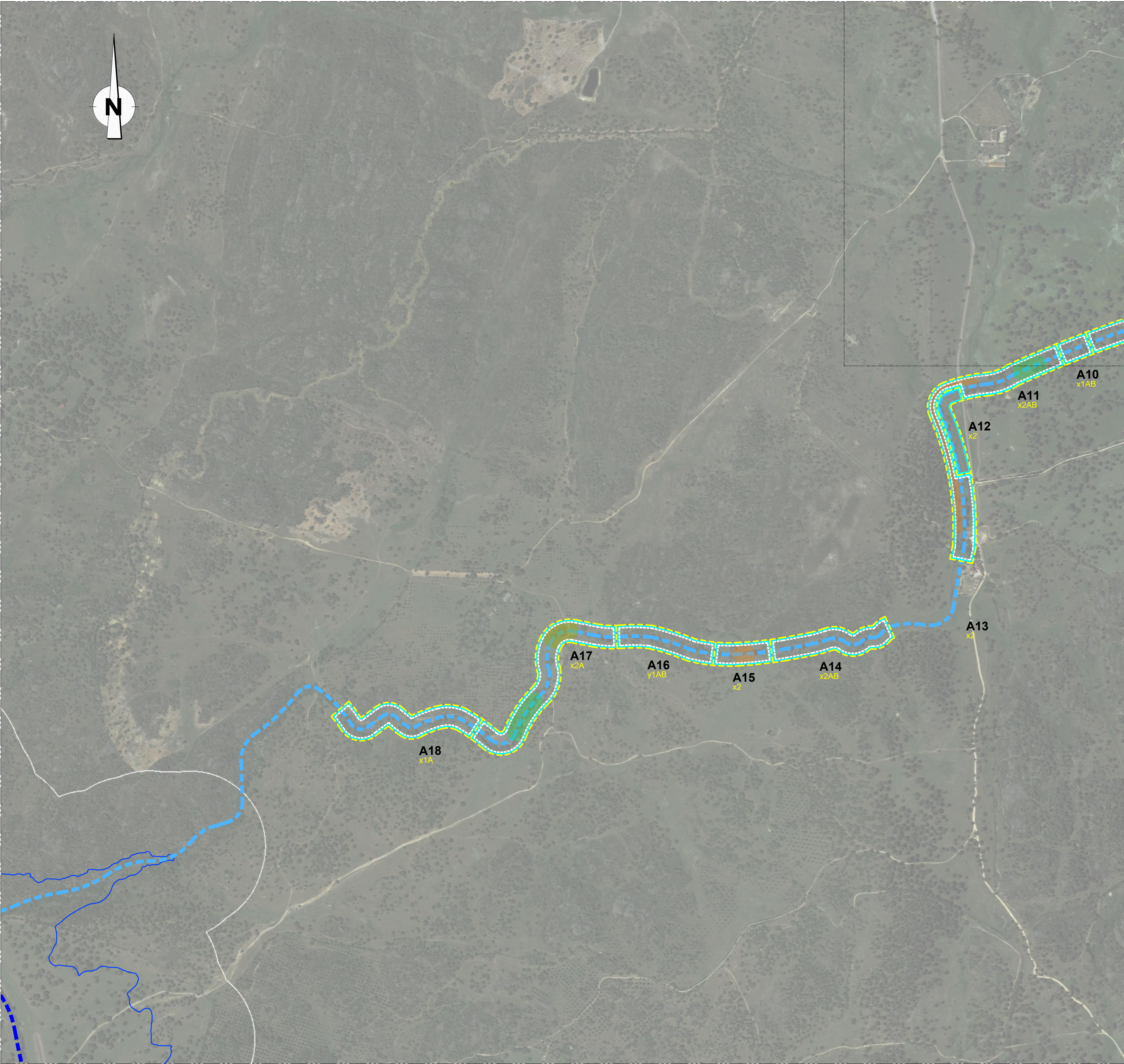
PLANTA - FOLHA 01 Esc. 1:5000
