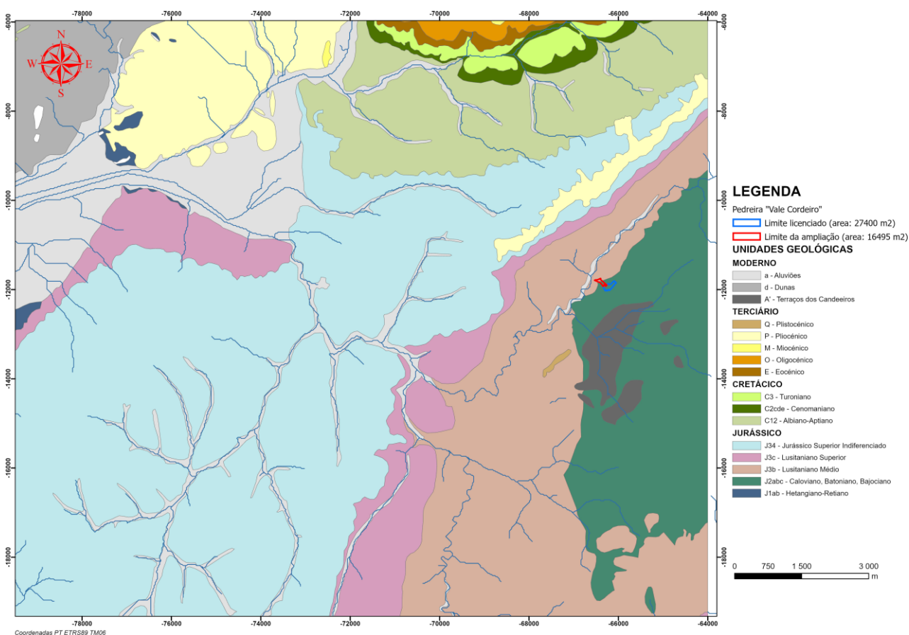
Figura 8 – Adaptação do extrato da Carta Geológica à escala 1/50000, com a localização da pedra.
