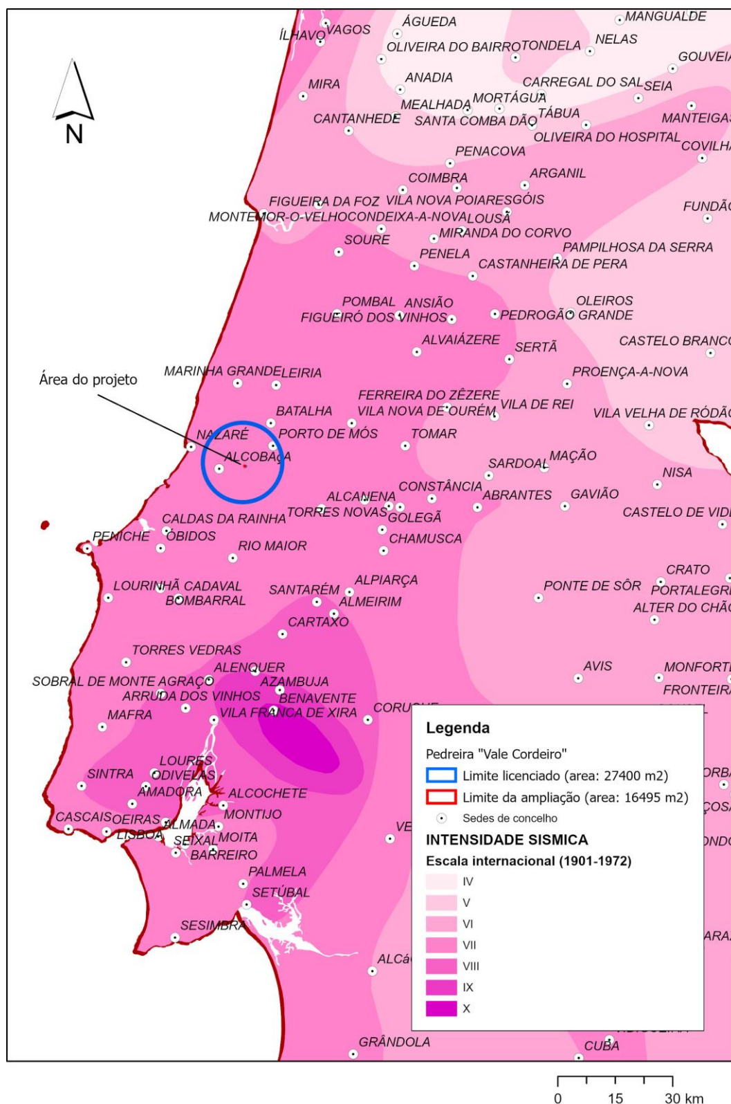
Figura 6 – Extrato da Carta de Intensidade Sísmica de Portugal, com a implantação da área do projeto.
