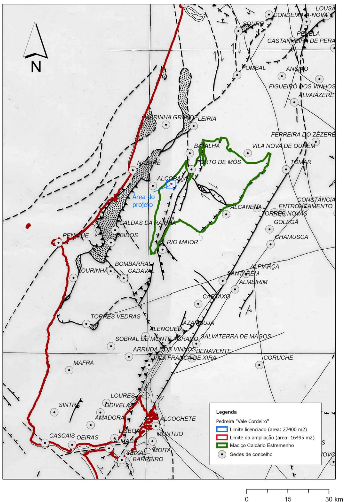
Figura 5 – Extrato da Carta Neotectónica de Portugal, com a implantação da área do projeto.
