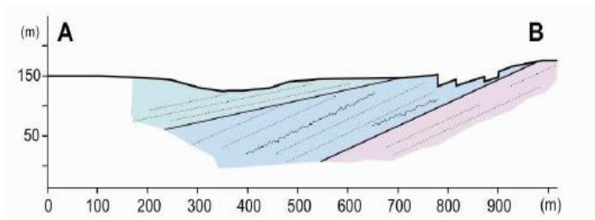
Figura 11 – Corte geológico esquemático do núcleo de pedreiras da Ataíja, na área afeta à pedreira “Vale Cordeiro N.º9 (Revista “A Pedra”, 2011).
