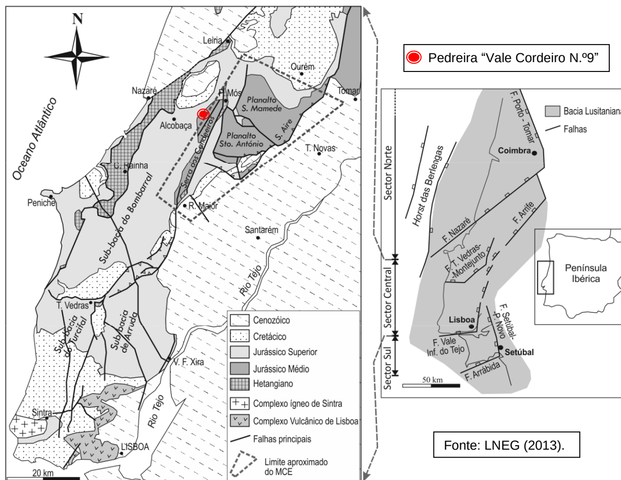
Figura 3 - Enquadramento do Maciço Calcário Estremenho no Setor Central da Bacia Lusitaniana (Subdivisões da Bacia Lusitaniana de acordo com Kullberg et al., 2006; geologia adaptada da Carta Geológica de Portugal à escala 1/1000000, ed. LNEG, 2011 (adaptado Carvalho, 2013).
