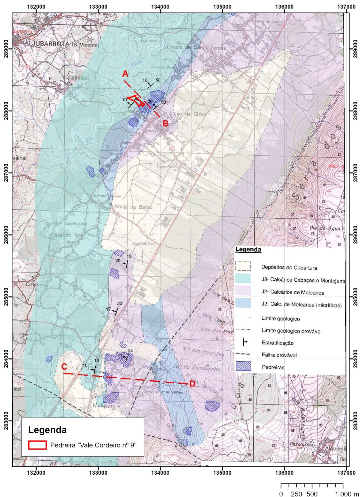
Figura 10 – Geologia da área da pedreira “Vale Cordeiro N.º9” (adaptado da revista “A Pedra”, 2011).
