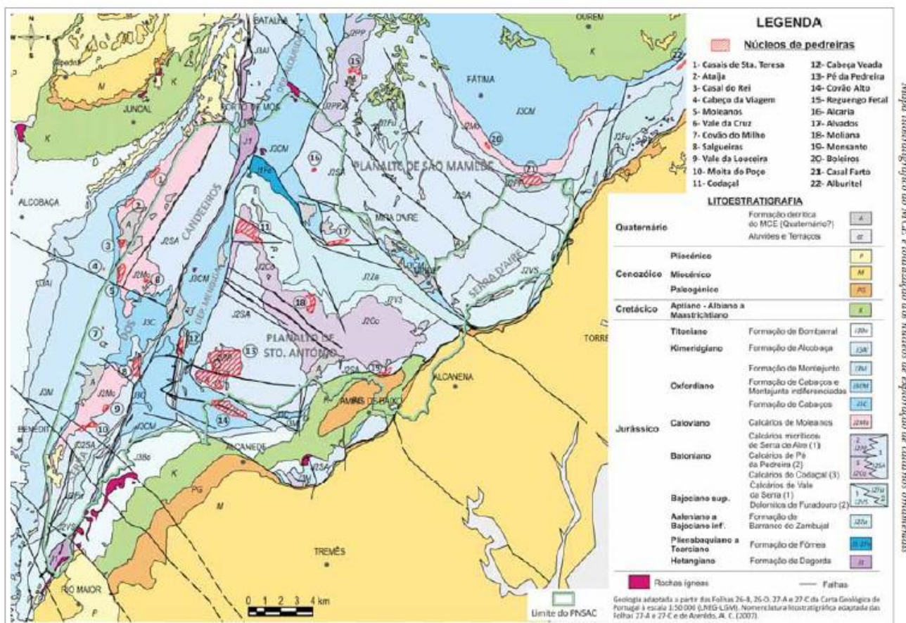
Figura 7 - Mapa litoestratigráfico do MCE e localização dos núcleos de exploração de calcários ornamentais (Fonte: Boletim de Minas, 47 (1), 2012).
