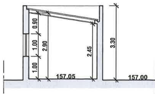
CORTE A-B
