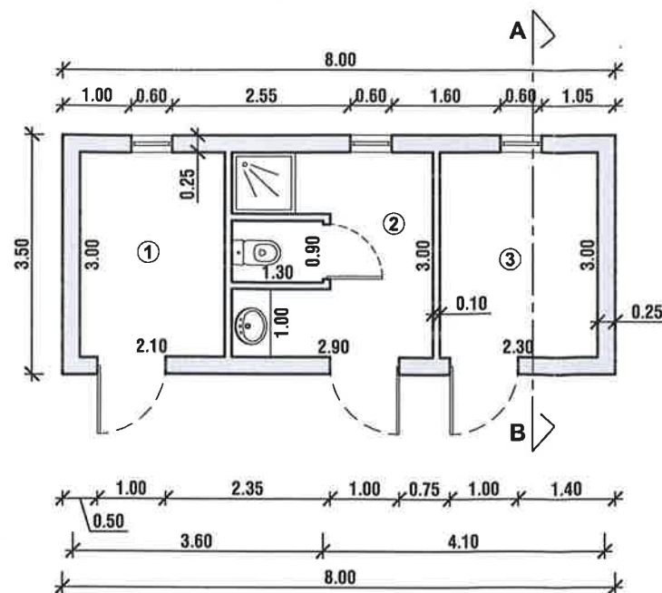
PLANTA DO PISO TÉRREO - ANEXO
