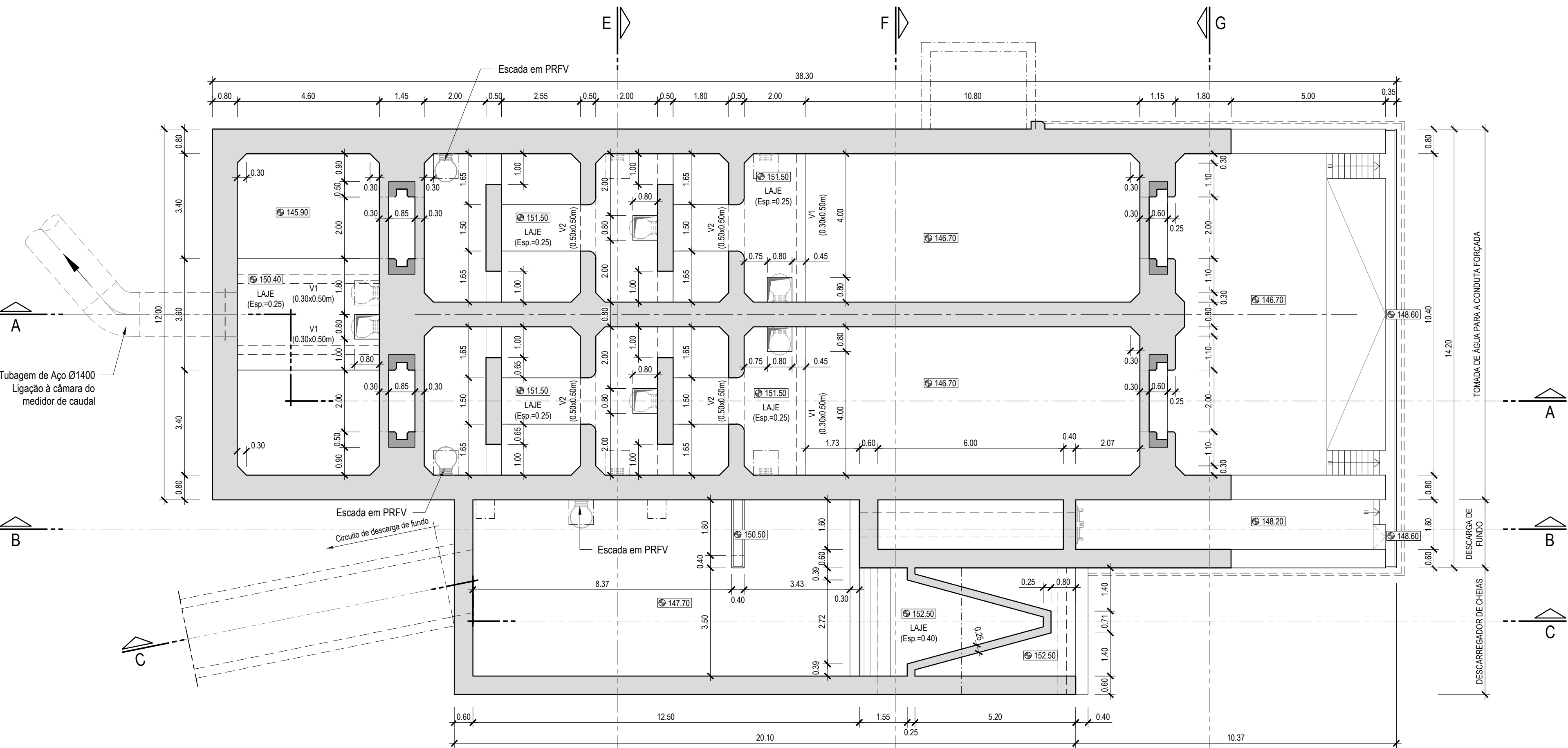
CORTE À COTA 153.00 Esc. 1:100
