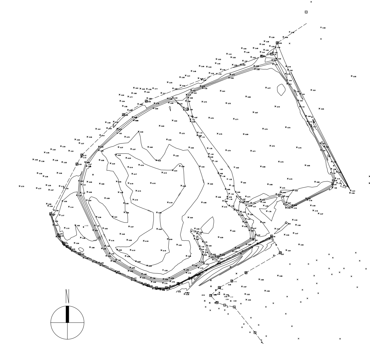
PLANTA TOPOGRÁFICA DO EXISTENTE 1:750
