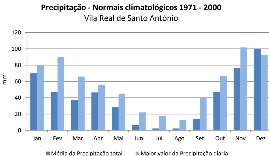
Figura 7. Evolução anual da precipitação média acumulada.
