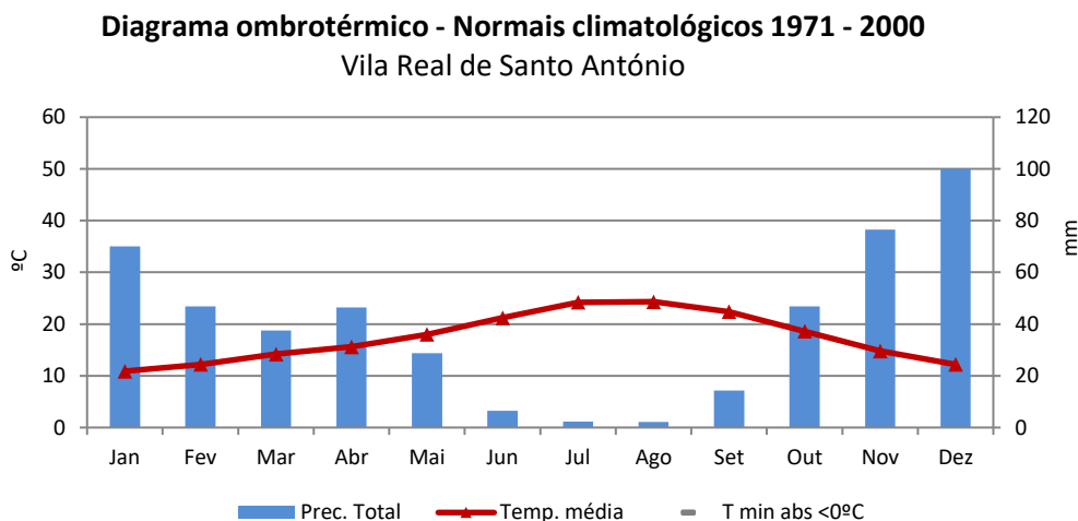
Figura 8. Diagrama ombrotérmico da área sob gestão.
