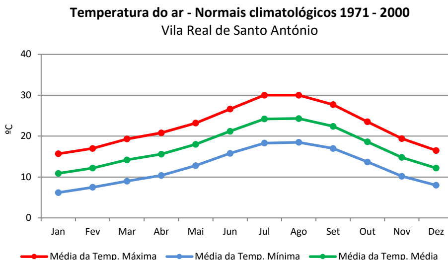
Figura 6. Evolução anual da temperatura média do ar.
