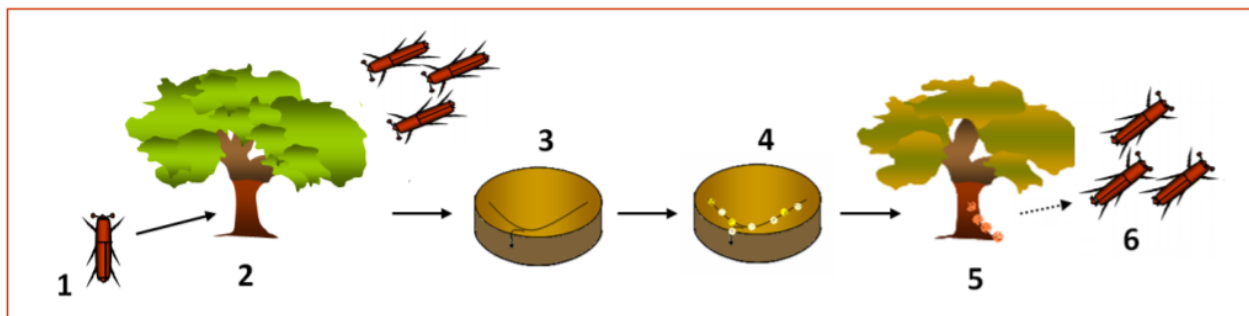
Figura 21. Esquema do ataque de Platypus cylindrus em sobreiro
