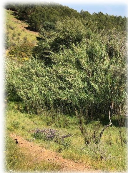
Figura 27. Canas observadas numa linha de água.
