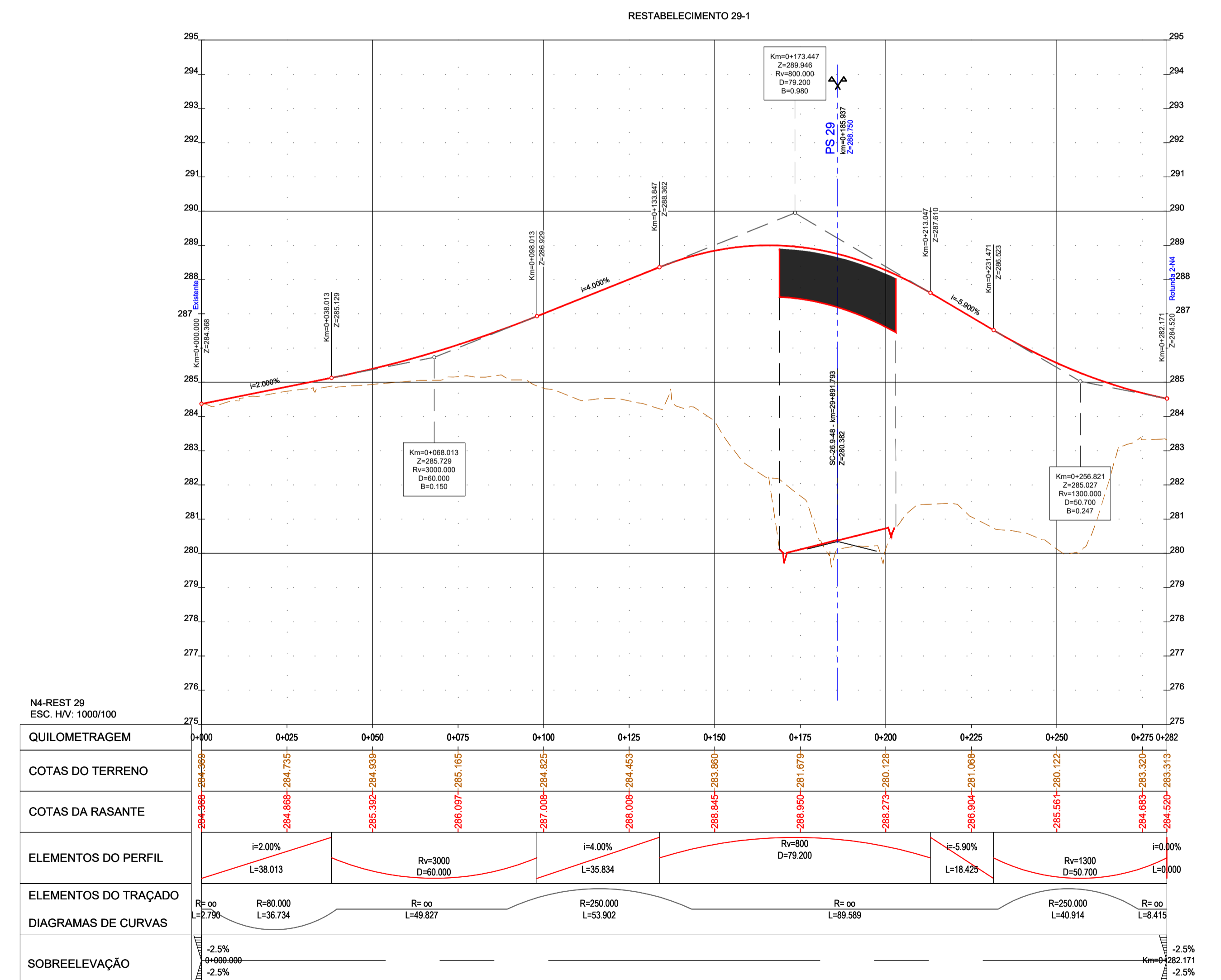
PERFIL LONGITUDINAL RESTABELECIMENTO 29-1 ESC. H= 1:1000 V= 1:100
