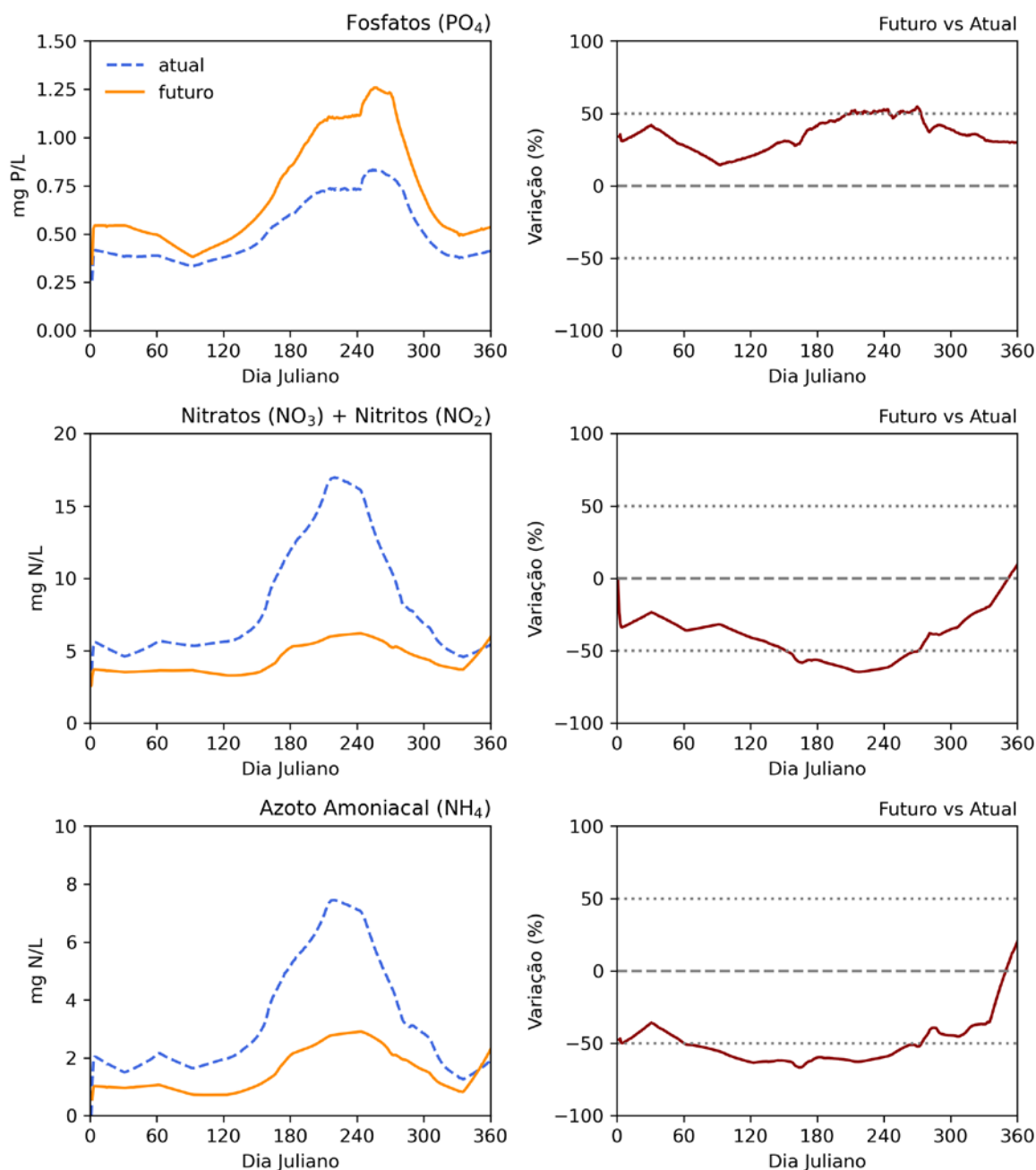
Figura 3.2 – Resultados do modelo para os cenários atual e futuro de parâmetros de qualidade da água - nutrientes.
