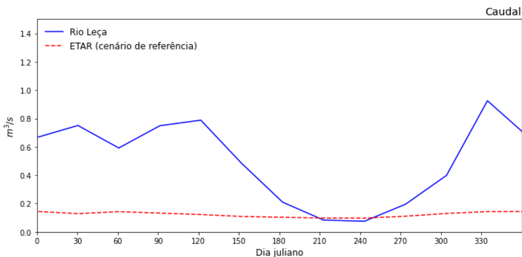
Figura 2.2 – Caudais utilizados para caracterizar o rio Leça e a descarga da ETAR (cenário de referência).
