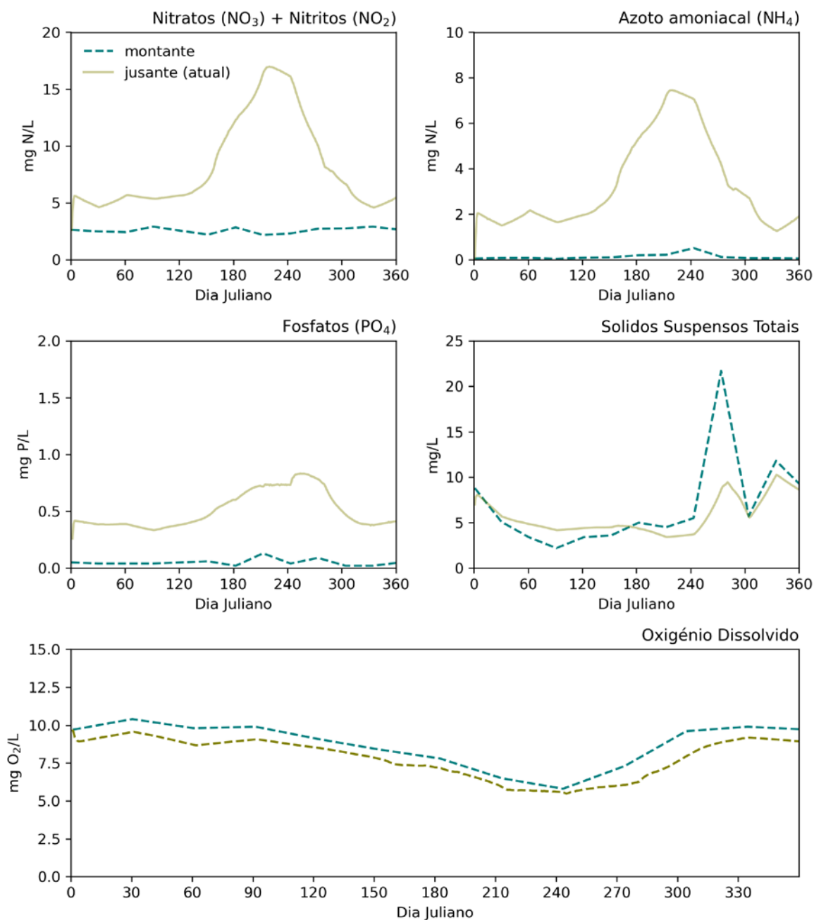
Figura 3.1 – Comparação das concentrações de parâmetros de qualidade da água a montante e a jusante da descarga da ETAR de Ermesinde e Alfena, no rio Leça. Os valores a montante foram obtidos através de dados da estação de qualidade do SNIRH, enquanto os valores a jusante correspondem às simulações do modelo, representando as condições atuais (situação de referência).
