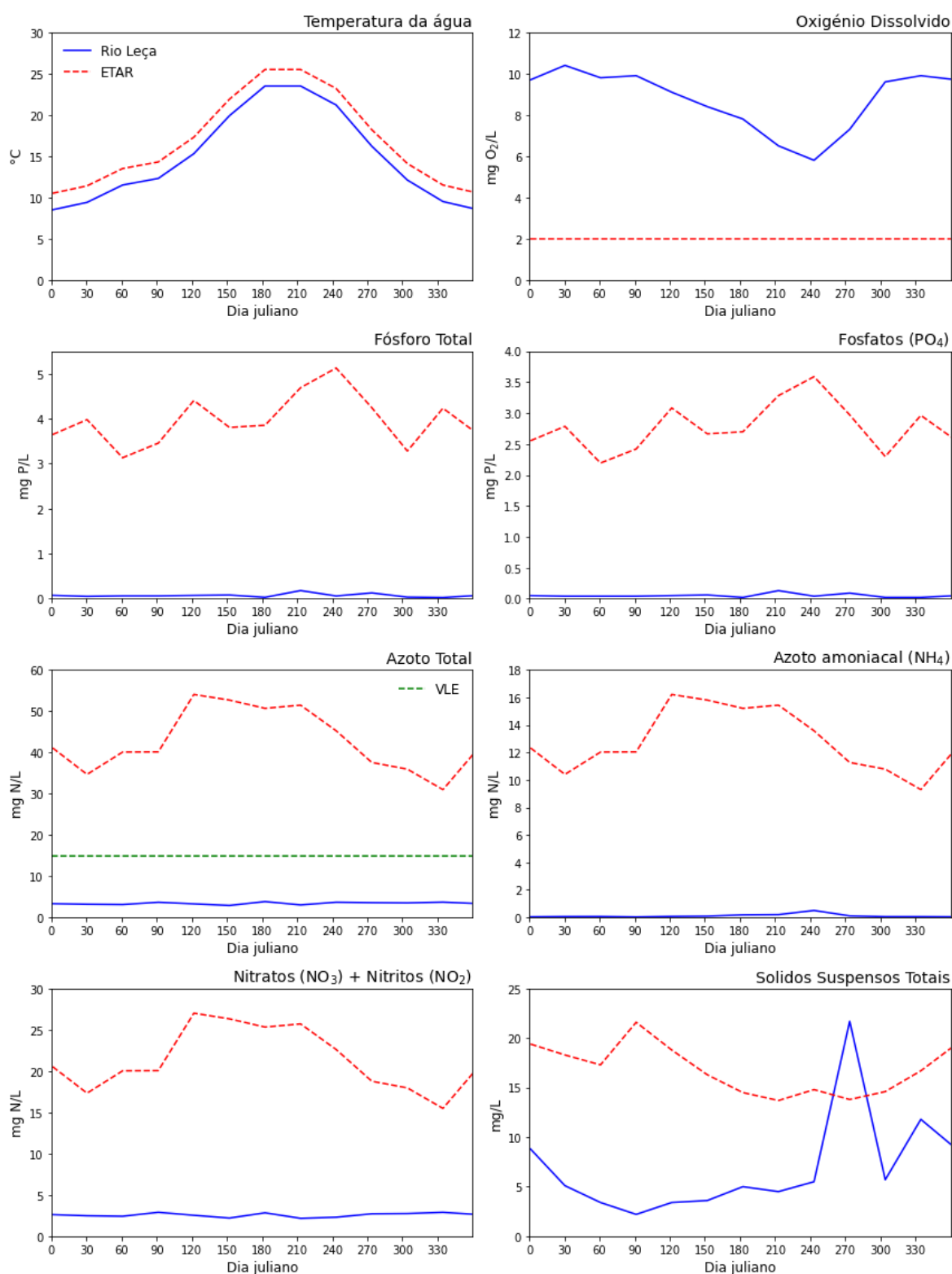
Figura 2.3 – Valores de entrada (médias mensais) dos parâmetros que caracterizam a qualidade da água do rio Leça e do efluente da ETAR de Ermesinde e Alfena.
