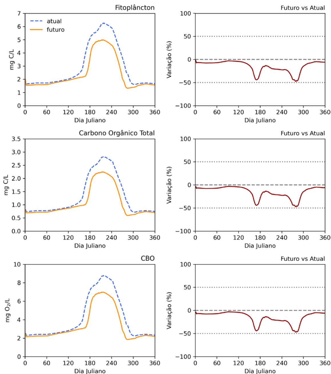
Figura 3.3 – Resultados do modelo para os cenários atual e futuro – fitoplâncton, COT e CBO.
