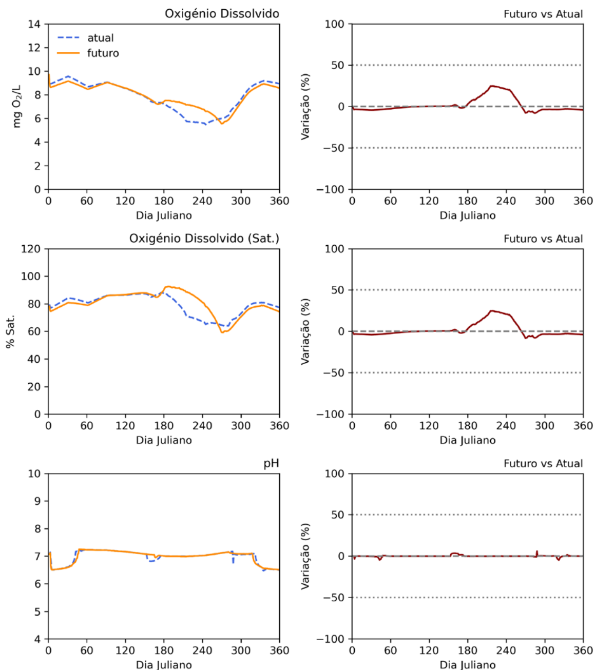
Figura 3.4 – Resultados do modelo para os cenários atual e futuro – OD e pH.
