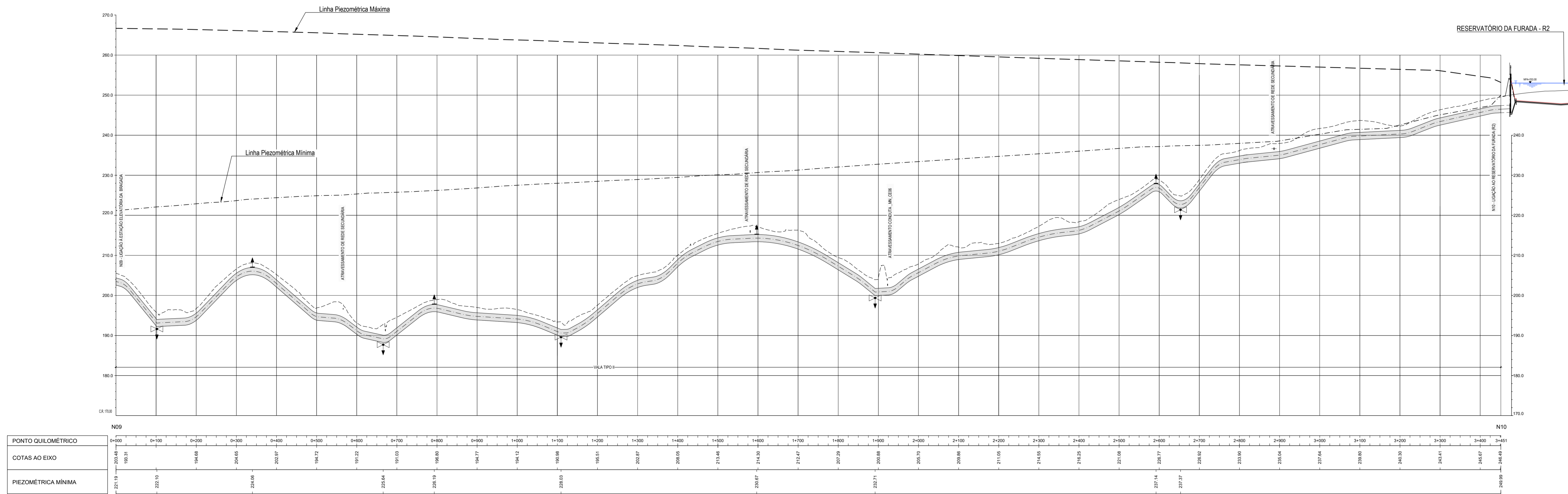
PERFIL LONGITUDINAL Esc. 1:5000(H) 1:5000(V)
