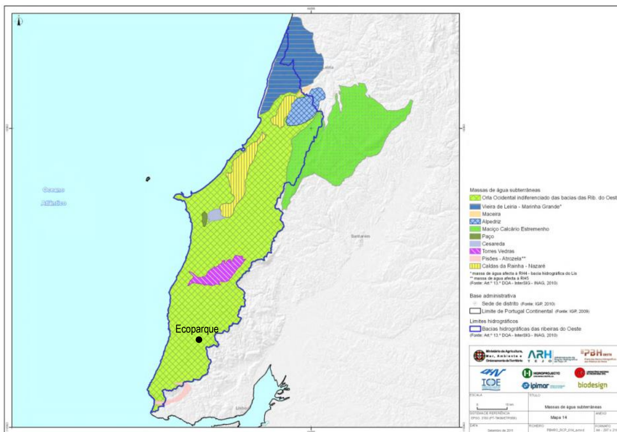
Figura 3.6 – Massas de águas subterrâneas na bacia hidrográfica das Ribeiras do Oeste
