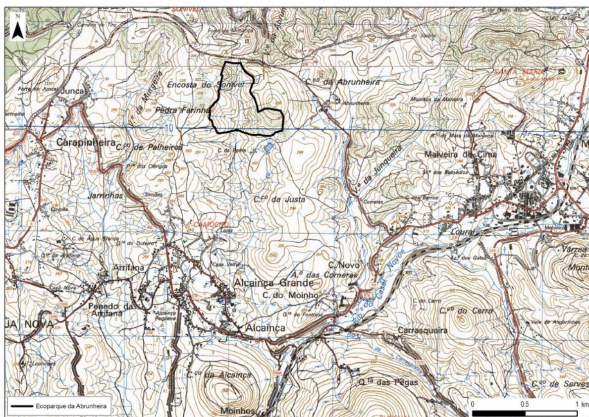
Figura 3.4 – Enquadramento hidrológico local Fonte: Carta Militar de Portugal, na escala 1:25000, Folhas 388 e 402
