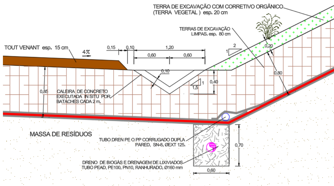
Figura Nº.31. - Caleira revestida em banquetas.
