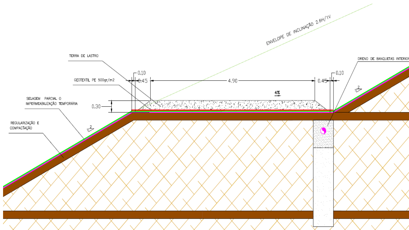
Figura 28 – Impermeabilizações temporárias na fase de exploração.
