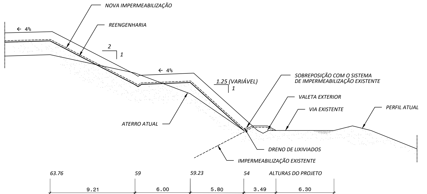
SEÇÃO "A". E: 1/200
