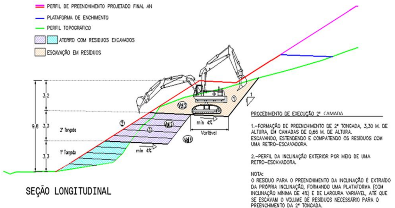
Figura 15. Fase-3 Sequência de perfilamento da inclinação de massa de resíduos atual
