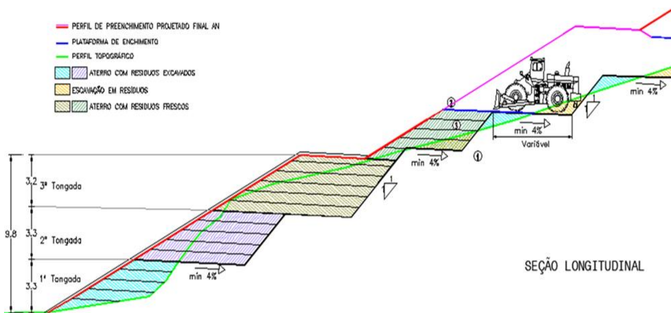
Figura 18. Avanço de perfilamento. Deposição de resíduos escavados e resíduos frescos.
