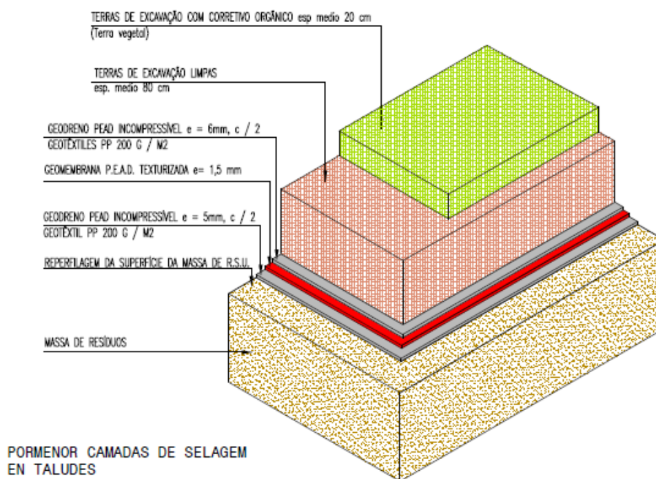
Figura 26. – Camadas de Selagem em Taludes
