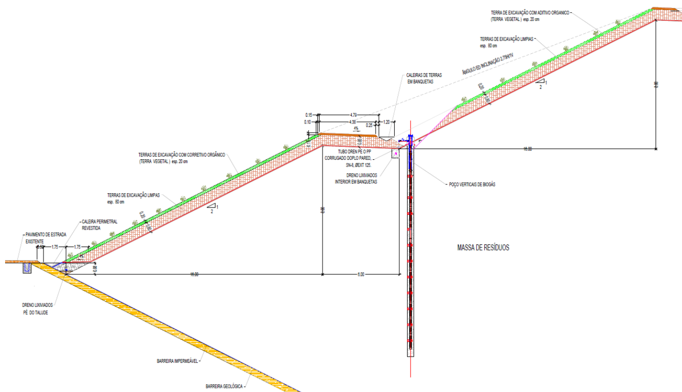
Figura 27. – Camadas de Selagem em Taludes
