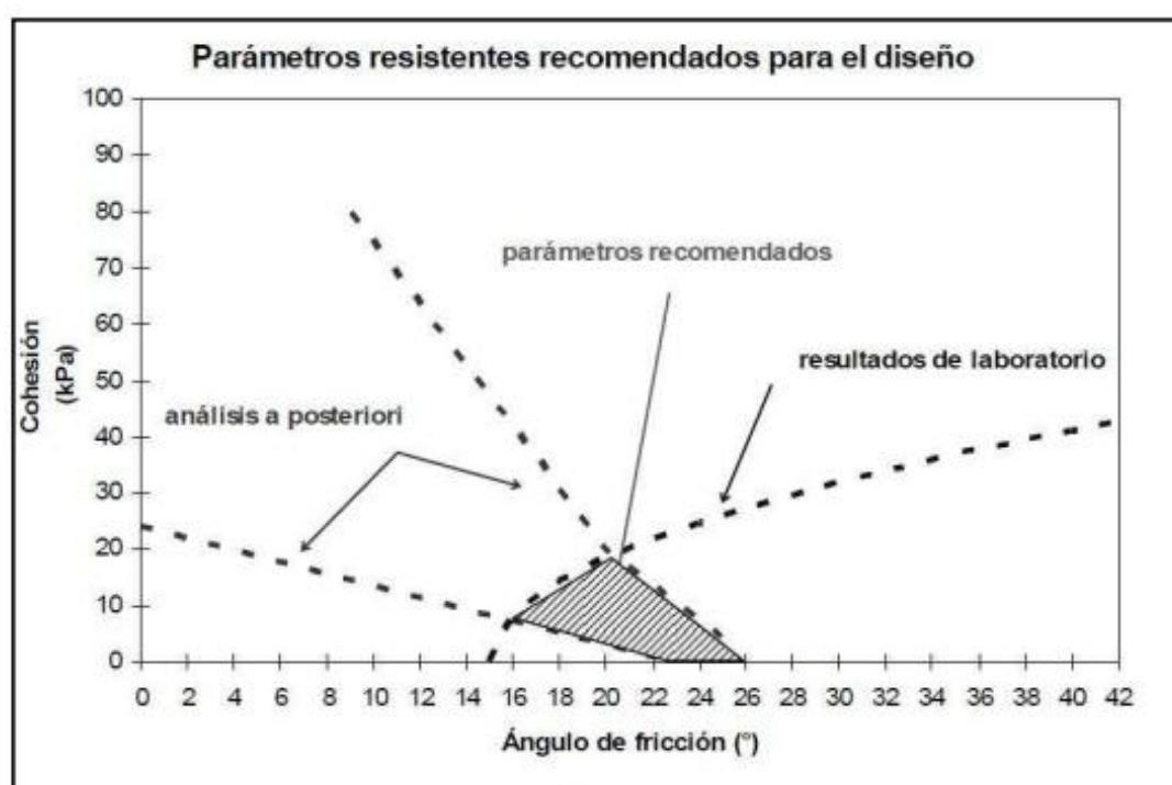
Figura 5 - Valores recomendados por Sánchez Alciturri et al, (1993).
