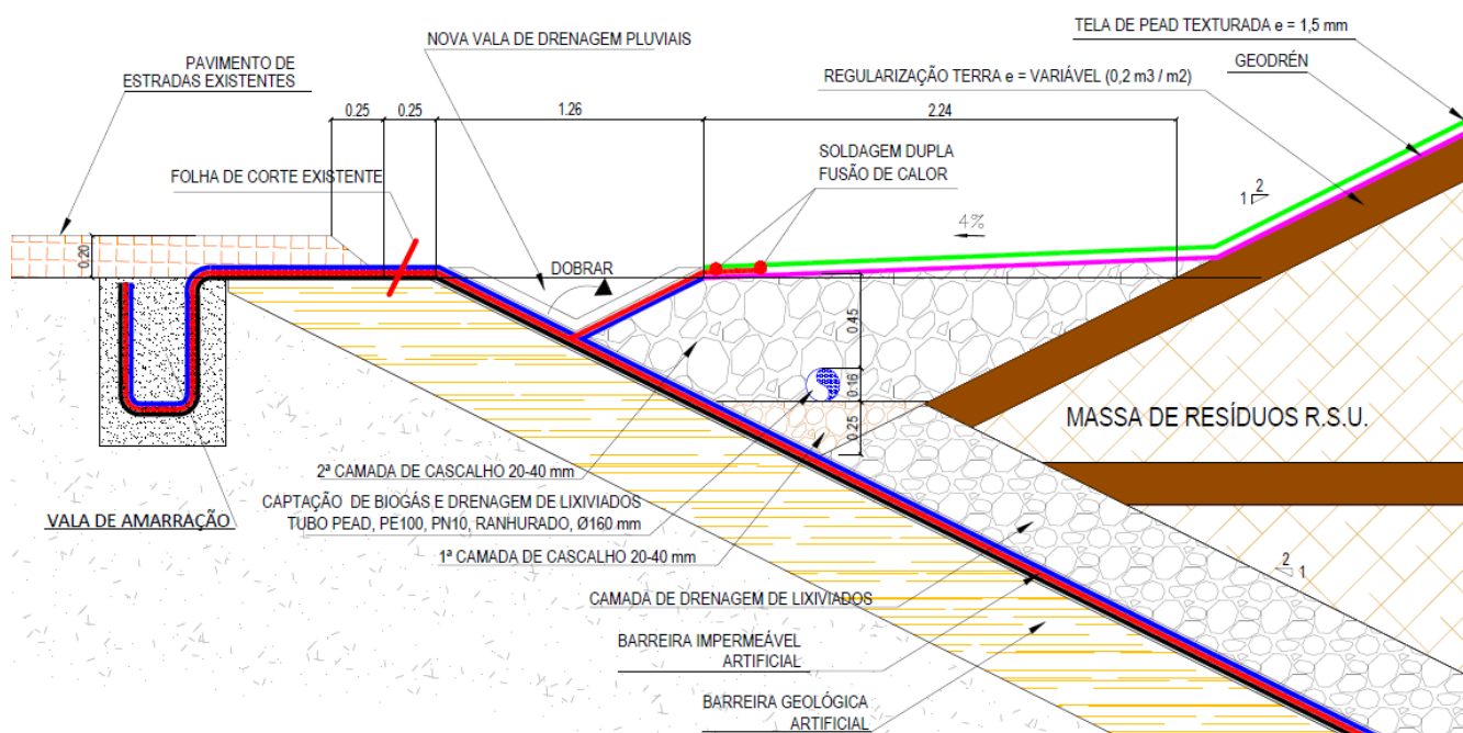
Figura 28 – Impermeabilizações temporárias na fase de exploração.
