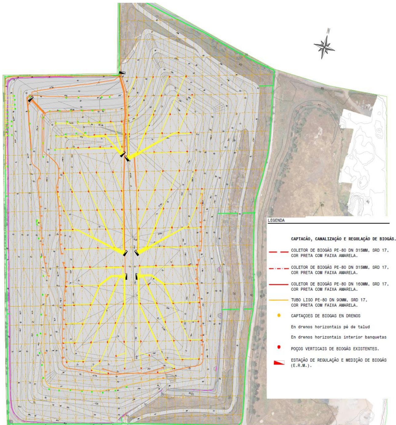
Figura 25— Desgaseificação planta geral.
