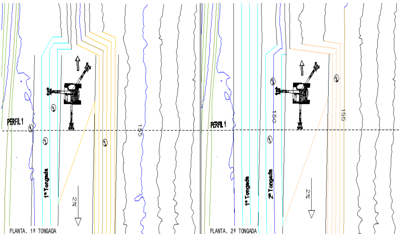
Figura 16. Sequência do avanço de perfilamento da inclinação de massa de resíduos, em diferentes níveis das banquetas.
