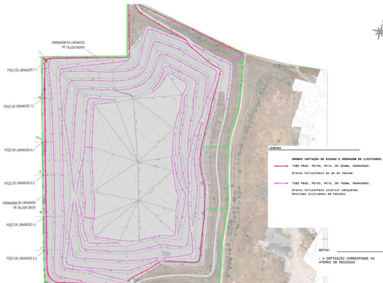
Figura 19. Drenagem de Lixiviados. Planta geral..
