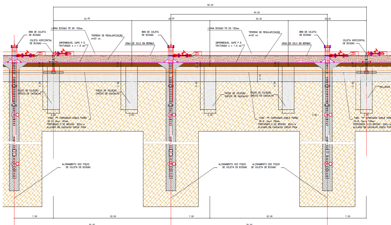
Figura 24– Detalhe de Poços Verticais de Biogás, interligados com os Drenos Horizontais.
