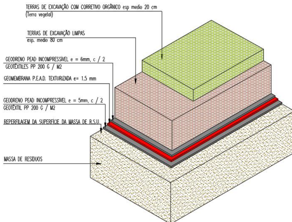
Figura 12 -Esquema camadas de Selagem
