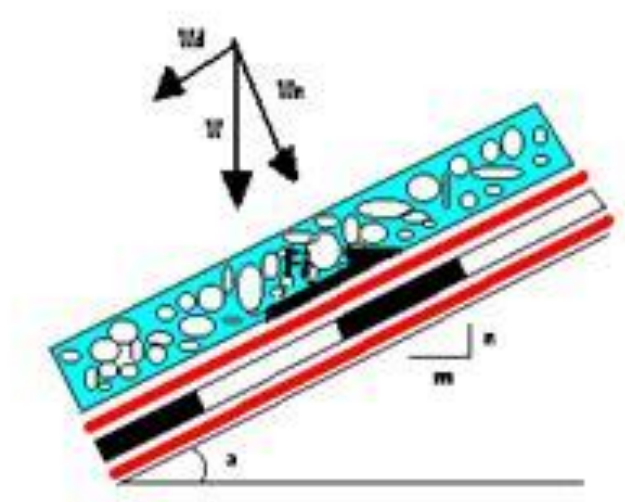
Figura 14 - Diagrama das forças que atuam no talude
