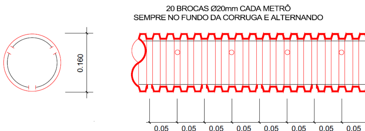
Figura 22– Seção Longitudinal da Rede de Lixiviados Intermédia das Banquetas.
