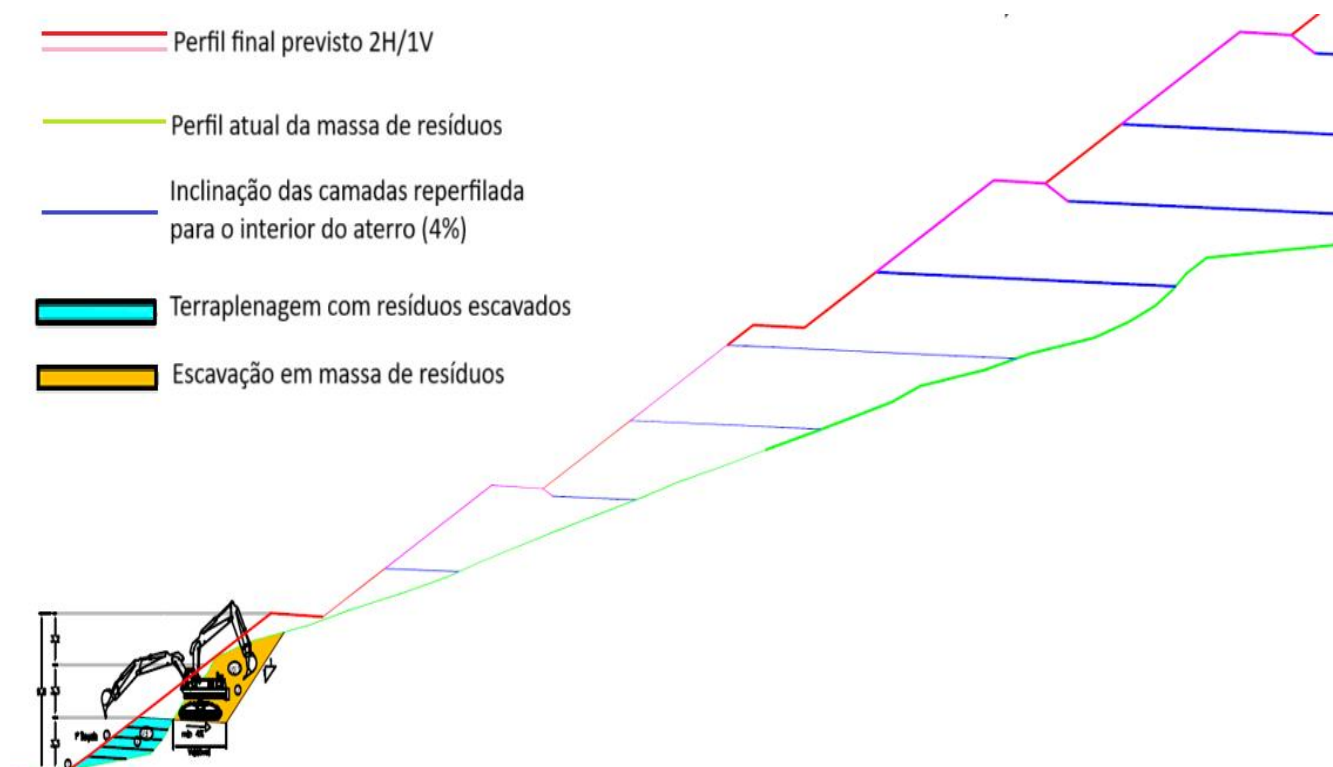
Figura 13. Fase-1 Sequência de reperfilamento da inclinação de massa de resíduos atual
