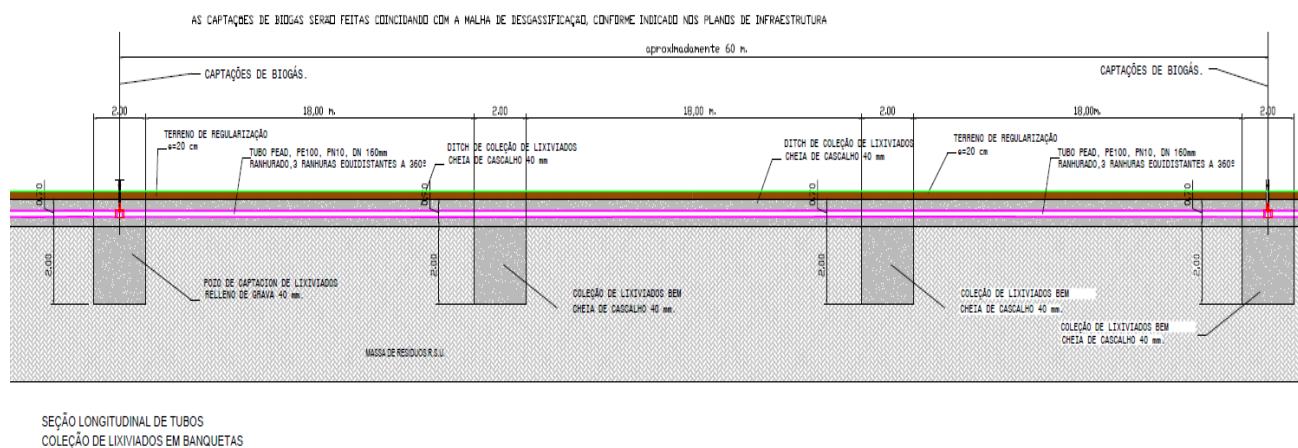
Figura 21– Secção Longitudinal da Rede de Lixiviados Intermédia das Banquetas.
