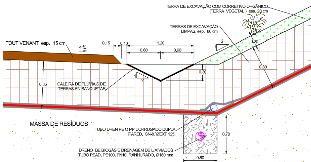
Figura Nº.30. - Caleira de terras em banquetas.
