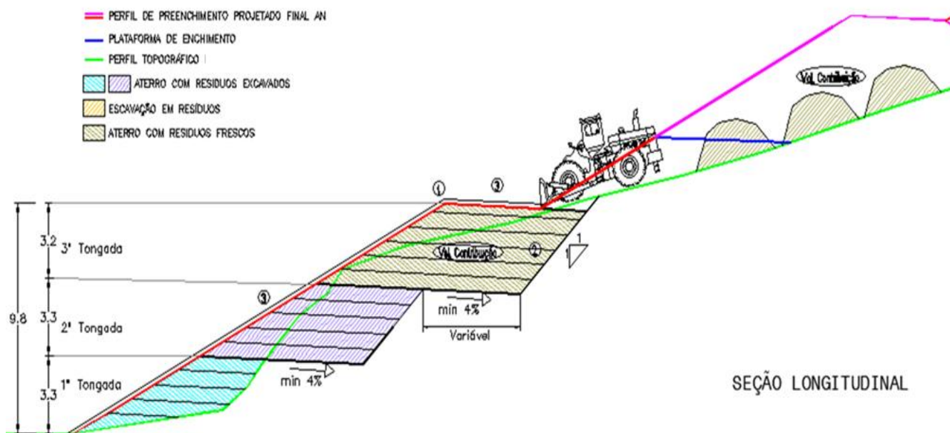
Figura 17. Avanço de perfilamento. Deposição de resíduos escavados.
