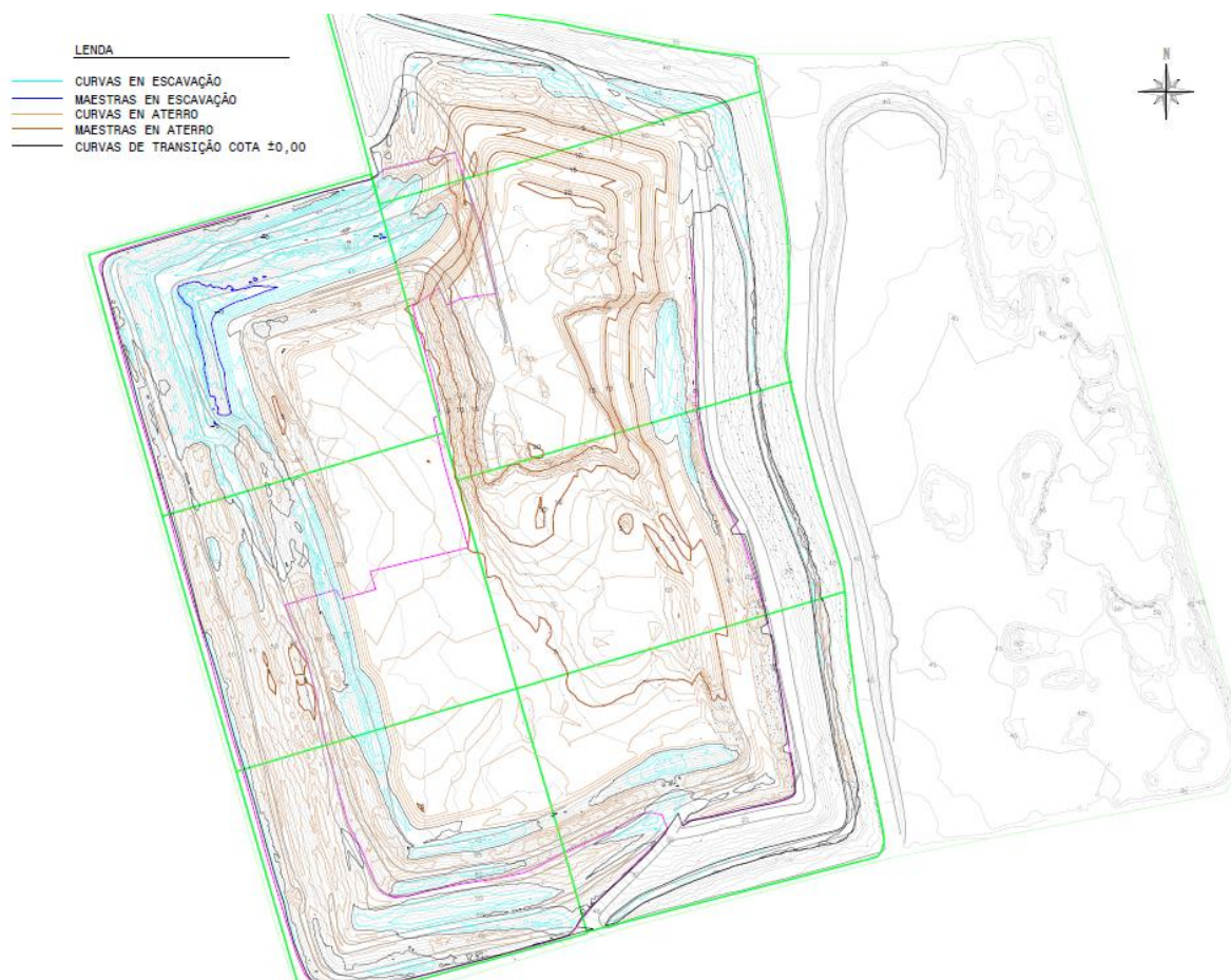
Figura 11.- Espessuras de escavação e terraplenagem das células 1 a 7 Aterro Palmela. Reperfilamento.
