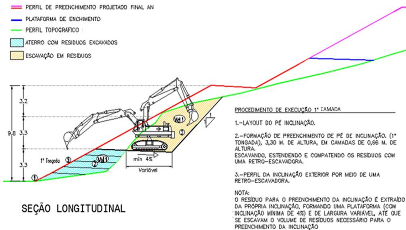
Figura 14. Fase-2 Sequência de perfilamento da inclinação de massa de resíduos atual
