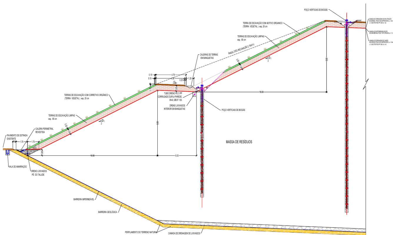
Figura 13 - Secção tipo. Selagem final
