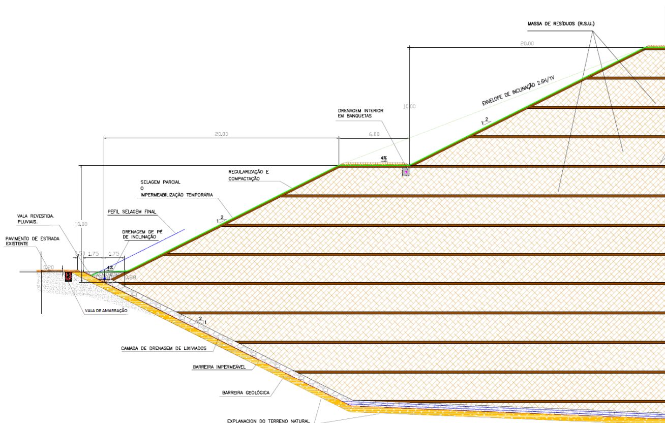
Figura 10.- Perfil tipo uma vez realizado o reperfilamento da massa de resíduos.
