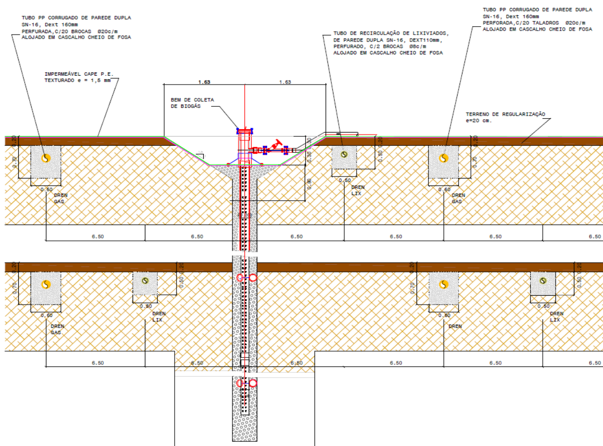
Figura 23— Secção Longitudinal da Rede de Lixiviados Intermédia das Banquetas.
