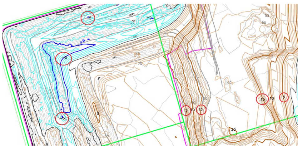
Figura 12.- Indicação do valor numérico da espessuras de escavação e terraplenagem do células 1 a 7 Aterro Palmela. Reperfilamento.
