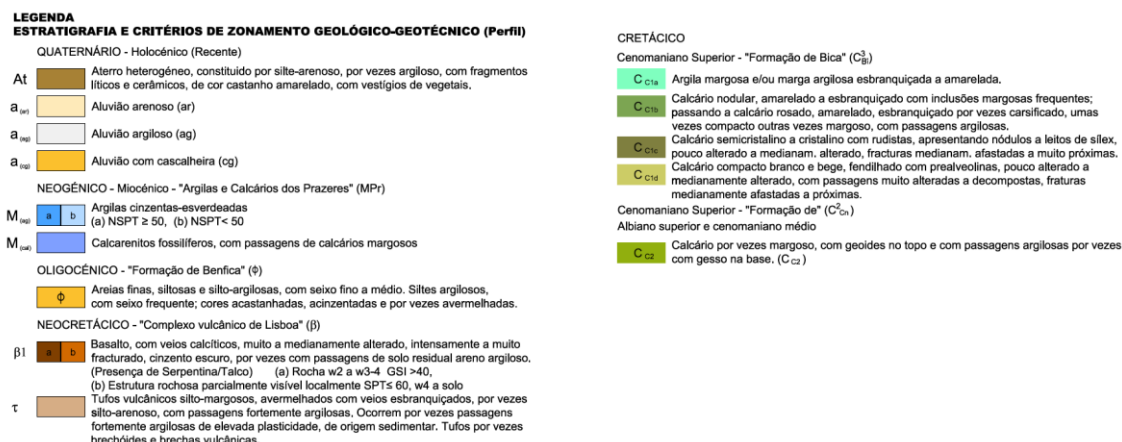
Figura 3 – Legenda das unidades representadas no Perfil longitudinal – Geologia / Geotecnia
