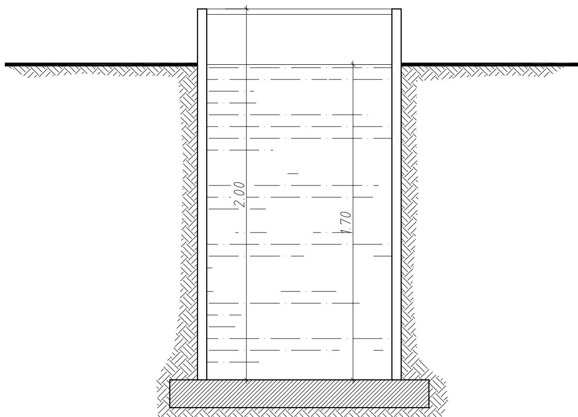
CORTE - FOSSA
