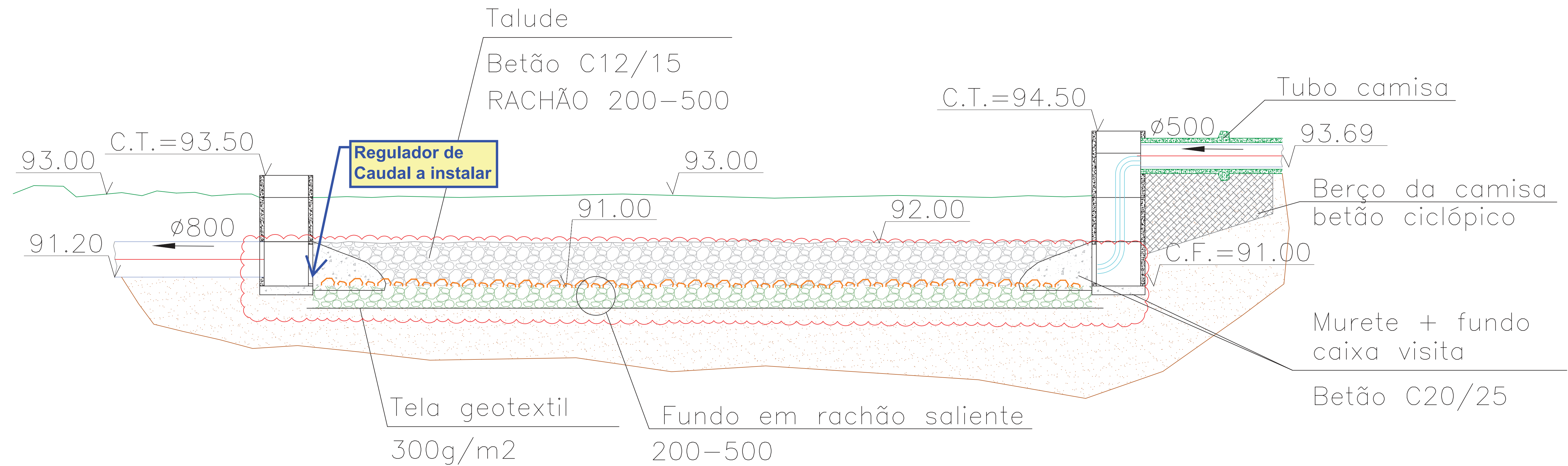
CORTE A-A
