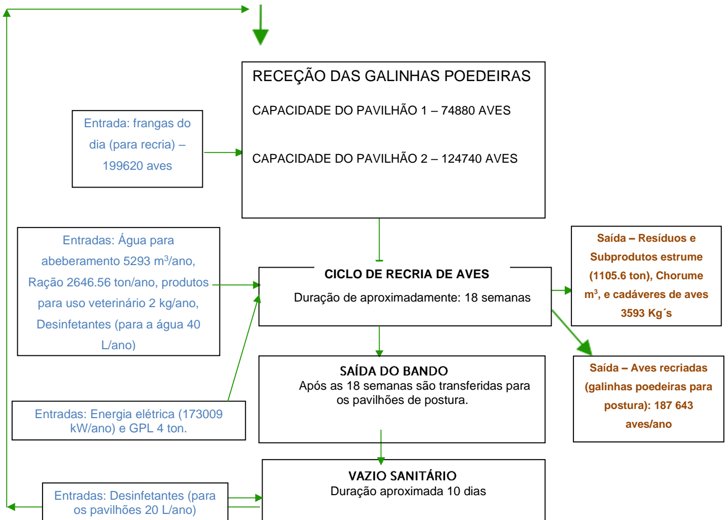
Figura 1 – Diagrama do processo de produção e balanço de massas
